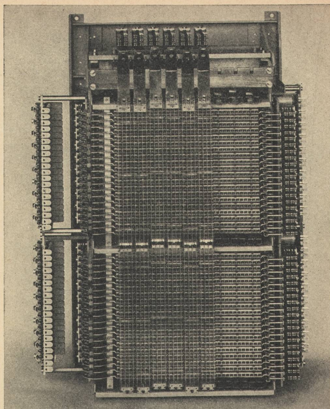
Kreuzwähler K 53
