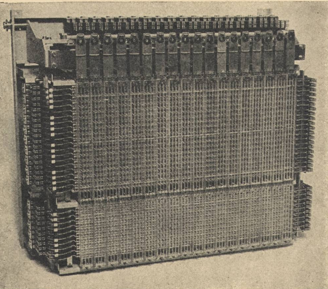
Kreuzwähler K 53
