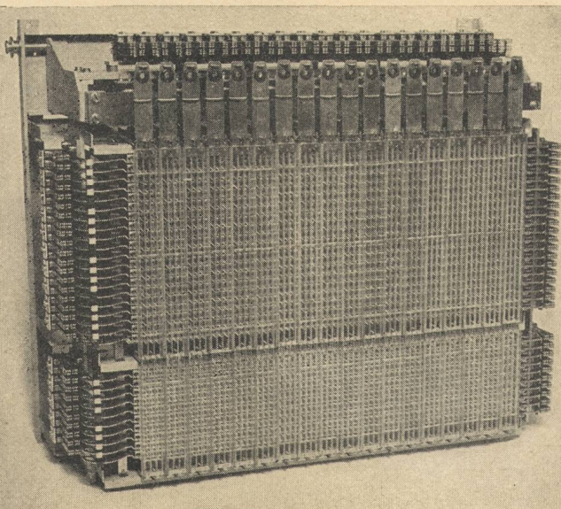
Kreuzwähler K 53
