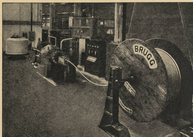
«Kontinuierliche Bleikabelpresse»
