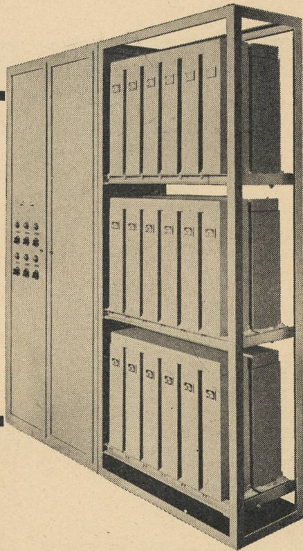
Automatische Blindstromkompensationsanlage, Blindleistung 240 kVar, Spannung 380 V \sim
