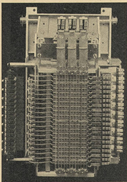
Kreuzwähler K53 zu Leitungsdurchschalter LD 19-3-0
