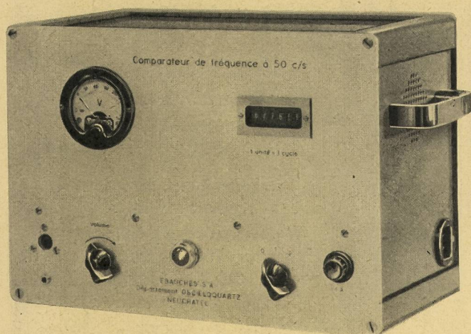
Comparateur de fréquence 50 c/s.
