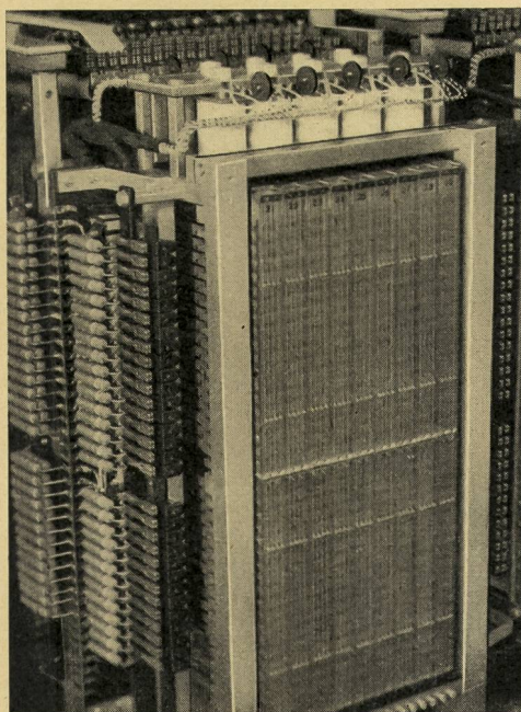
Kreuzwähler eines Telephonauten
