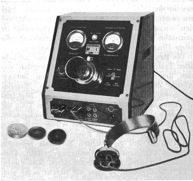
Fig. 1. Mikrofonkapsel-Prüfgerät Appareil d'essai pour capsules microphoniques
