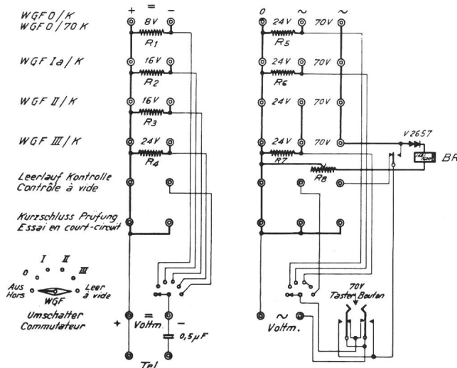
Fig. 8. Widerstandskasten für die Belastungsprüfung von Speisegleichrichtern, WGF-Typen
