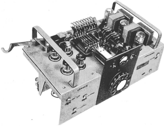
Fig. 6. Apparate-Chassis der Teilnehmerstation Châssis d'appareils de la station d'abonné
