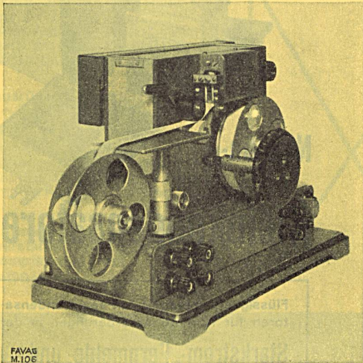
Registrierchronograph Typ M-427
