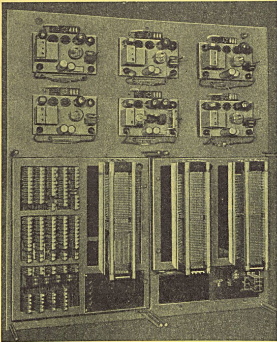
Automatische Wähleinrichtung für eine Gegensprechanlage
