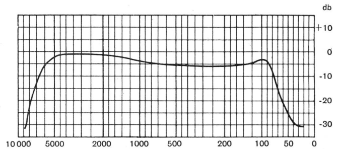
Fig. 7. Totale Frequenzcharakteristik. Caractéristique de fréquences totale.
