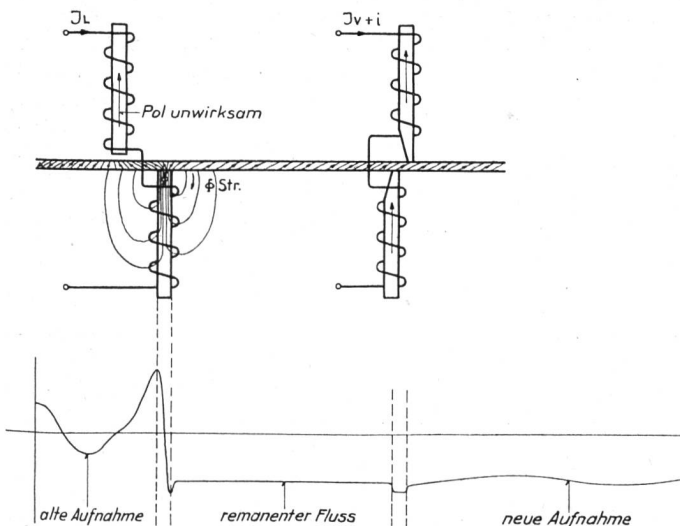
Fig. 8. Vorgang bei falschem Löschen. — Erreur d'effacement.
