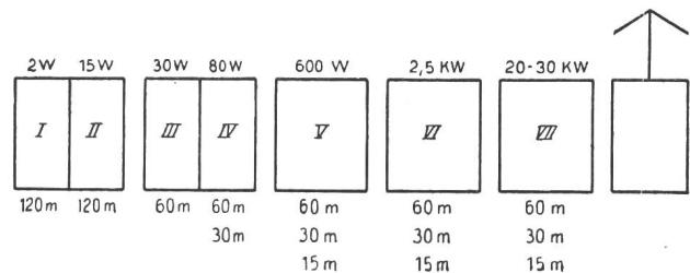
Fig. 7b. Stufenschema für statisch stabilisierte Kurzwellen-Grosssender (Telefunken). Schéma des émetteurs d'ondes courtes à grande puissance, type Telefunken, à stabilisation statique.
