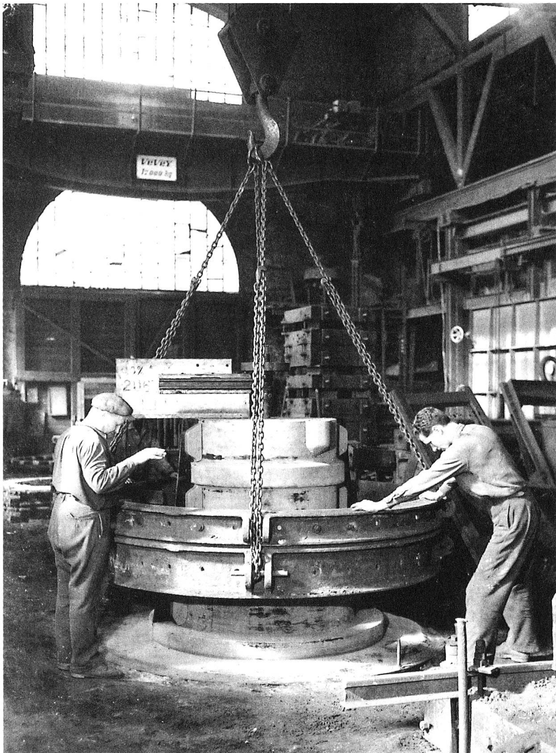
Ci-dessus: Deux ouvriers occupés auprès d'une turbine « Kaplan » en 1948 (négatif 9 x 12 N° 1899, Studio-reportage Edouard Curchod, Vevey).
