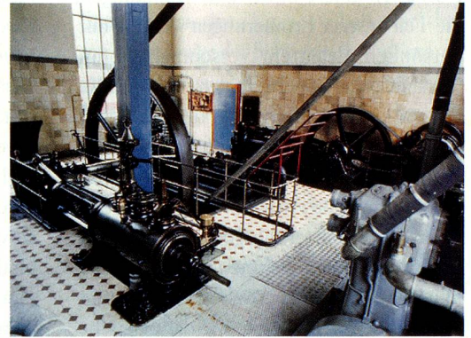
Uster, 1980: Sudkessel in der Brauerei Uster mit der letzten Dampfmaschine des Zürcher Oberlands. Die Ventilmaschine und der Kältekompressor stammen von 1897
