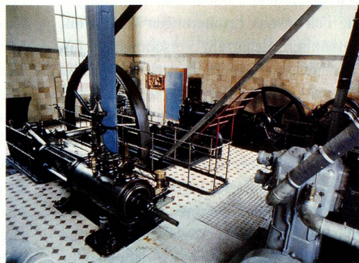
Uster, 1980: Sudkessel in der Brauerei Uster mit der letzten Dampfmaschine des Zürcher Oberlands. Die Ventilmaschine und der Kältekompressor stammen von 1897
