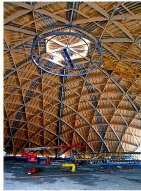
Riburg, 2005: Logistik- und Lagerzentrum der Rheinsalinen mit einer 31 Meter hohen Holzkuppel
