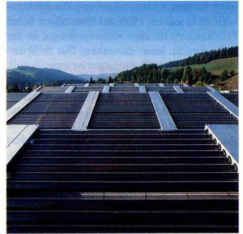
Weltweit einmalig: Schweizer Teigwarenfabrik erzeugt mittels einer Solaranlage auf dem Dach (Bild) Prozesswärme. (Foto: pd)
