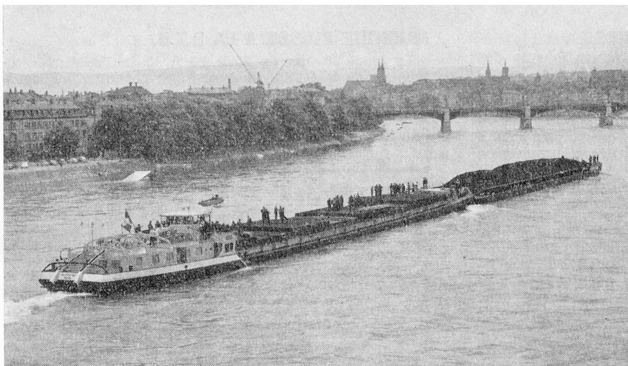
Automoteur poussant BLUEMLISALP, capacité 1500 t/1800 CV avec l'allège poussée BRAG 21, capacité 1700 t. Longueur totale 158 m. Capacité de transport totale avec 2 bacs : 4900 t.
