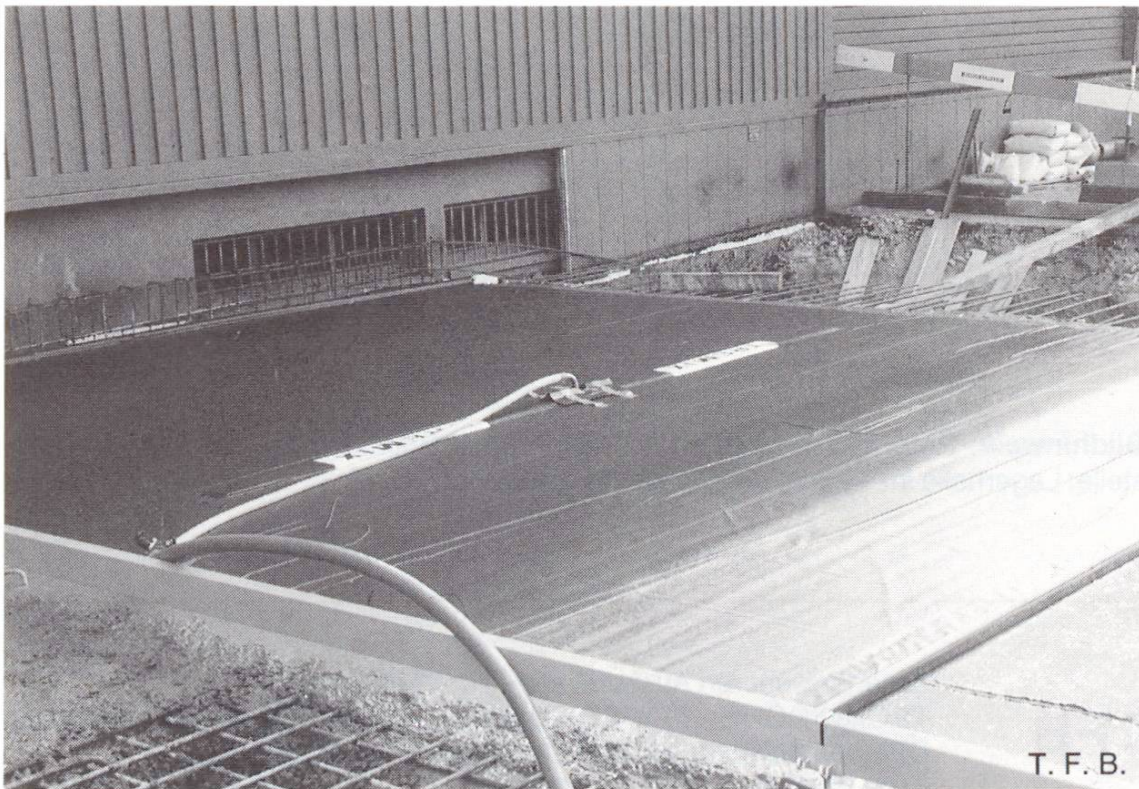
Abb. 2 Vakuumbehandlung.
