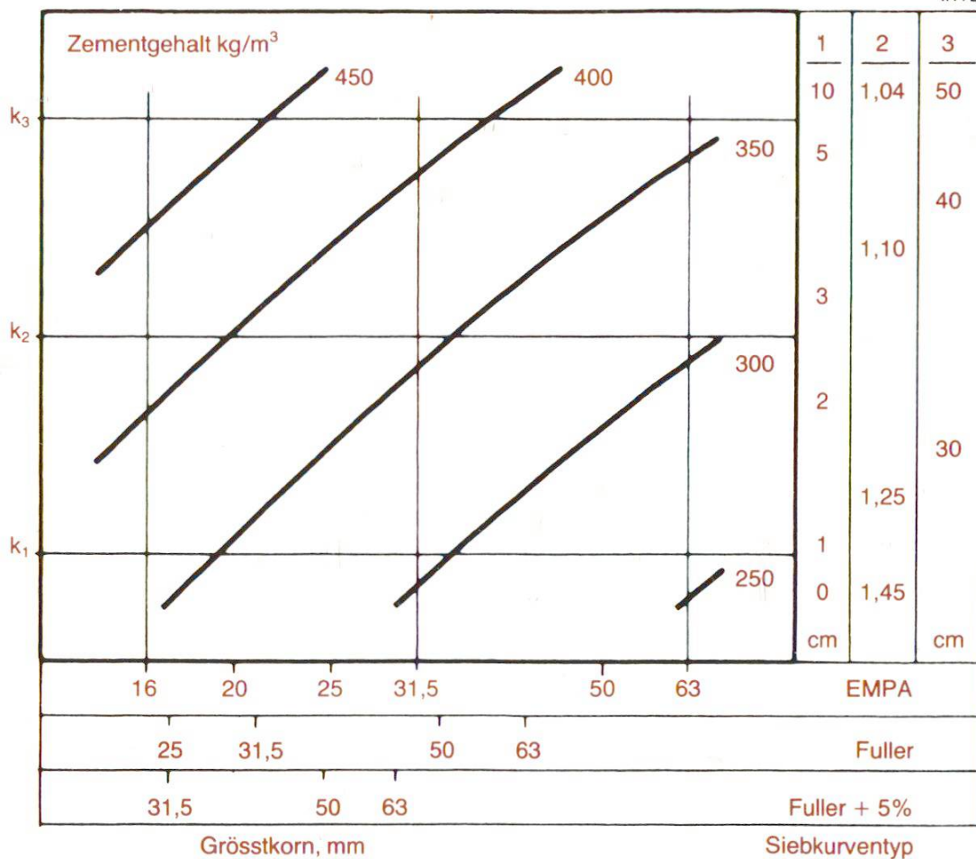
Abb. 3 Für Beton mit 55 \text{ N/mm}^2 nach 28 Tagen – mittlere Würfeldruckfestigkeit.
