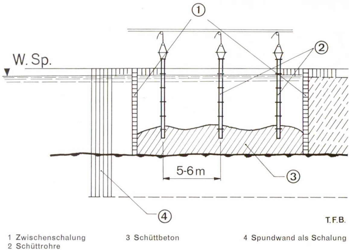
Abb. 4 Schematische Darstellung des Kontraktor-Verfahrens.
