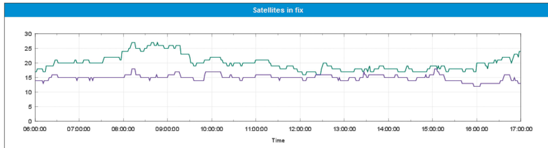
Abbildung 2: Vergleich Mountpoints am 18.09.2019 GPS/GLO (RTCM 3.1) und GPS/GLO/ GAL/BDS (RTCM 3.2 MSM)
