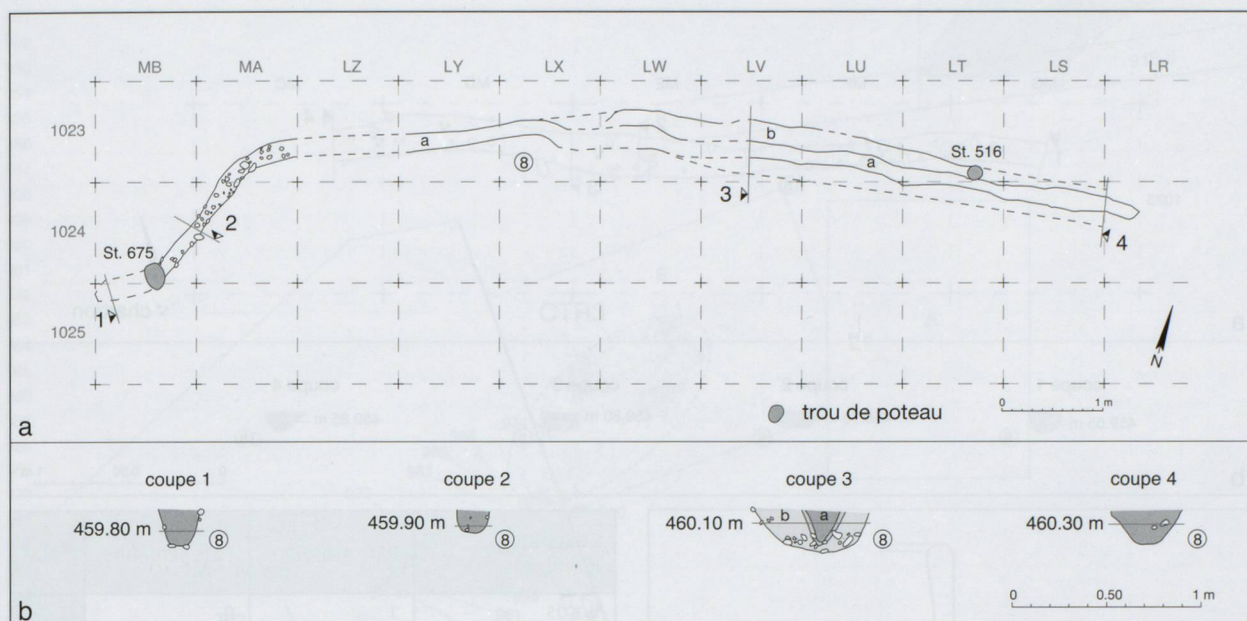
Fig. 46. Onnens-Le Motti. Plan (a) et coupes (b) de la structure St. 507. La couche 8 renvoie à la coupe de référence présentée au chapitre 2.2, p. 31.
