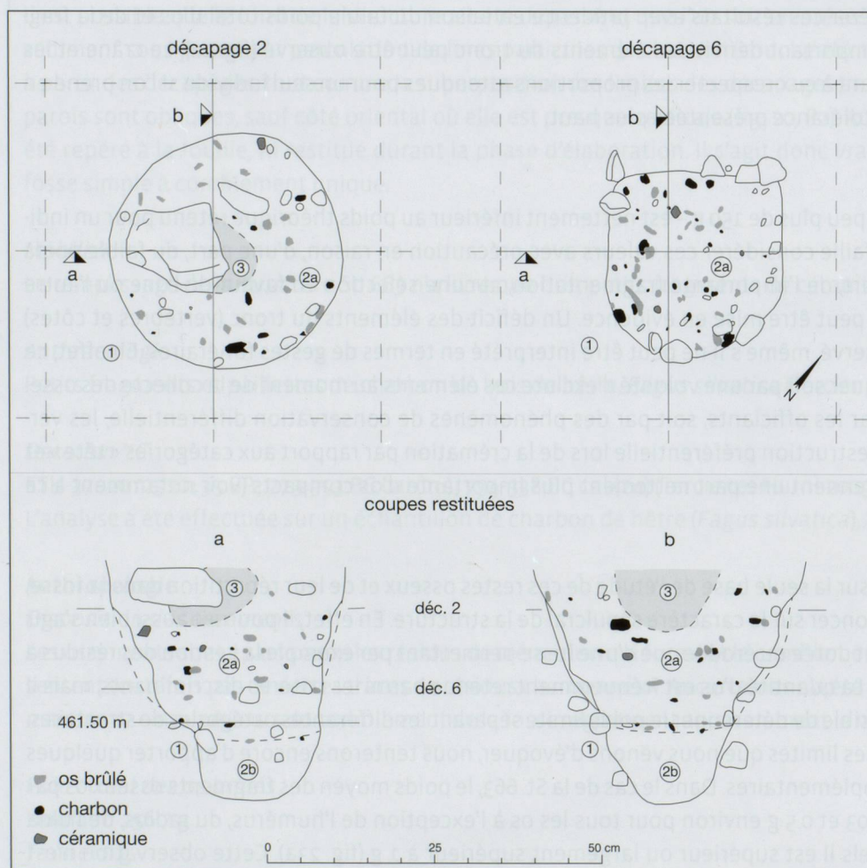
Fig. 20. Onnens-Le Motti. St. 663: plans (décapages 2 et 6) et coupes restituées. Les couches 1, 2 et 3 sont décrites dans le texte de présentation de la structure.
