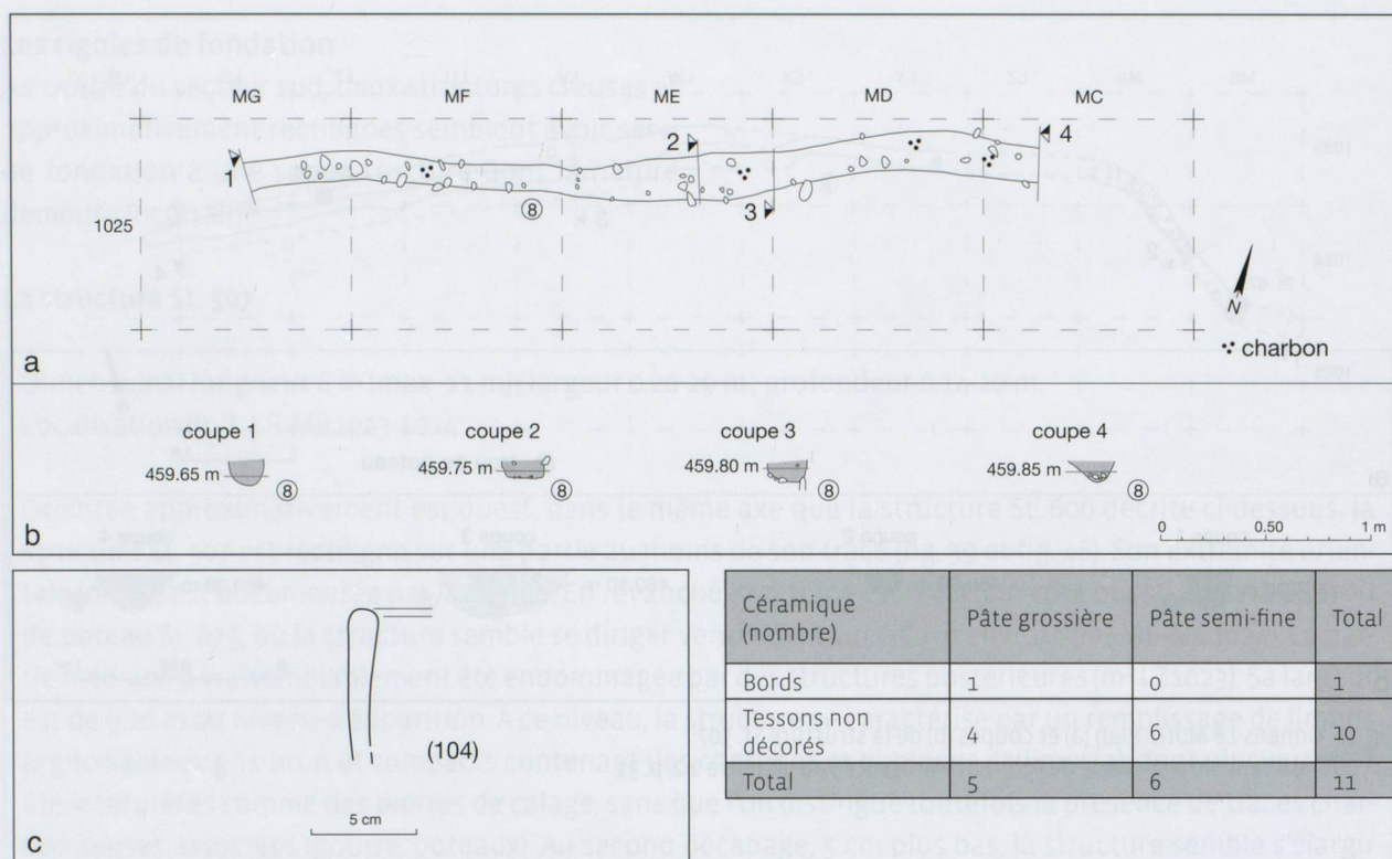
Fig. 47. Onnens-Le Motti. Plan (a), coupes (b), mobilier (c) et tableau synthétique du mobilier céramique de la structure St. 600 (d). La couche 8 renvoie à la coupe de référence présentée au chapitre 2.2, p. 31.
