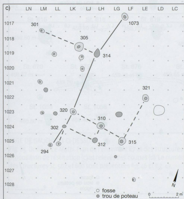
Fig. 84. Onnens-Le Motti. Plan de l'ensemble E6 et des structures associées avec (a) et sans (b) indication du numéro des structures; proposition de restitution (c) et relevés des coupes (d).
