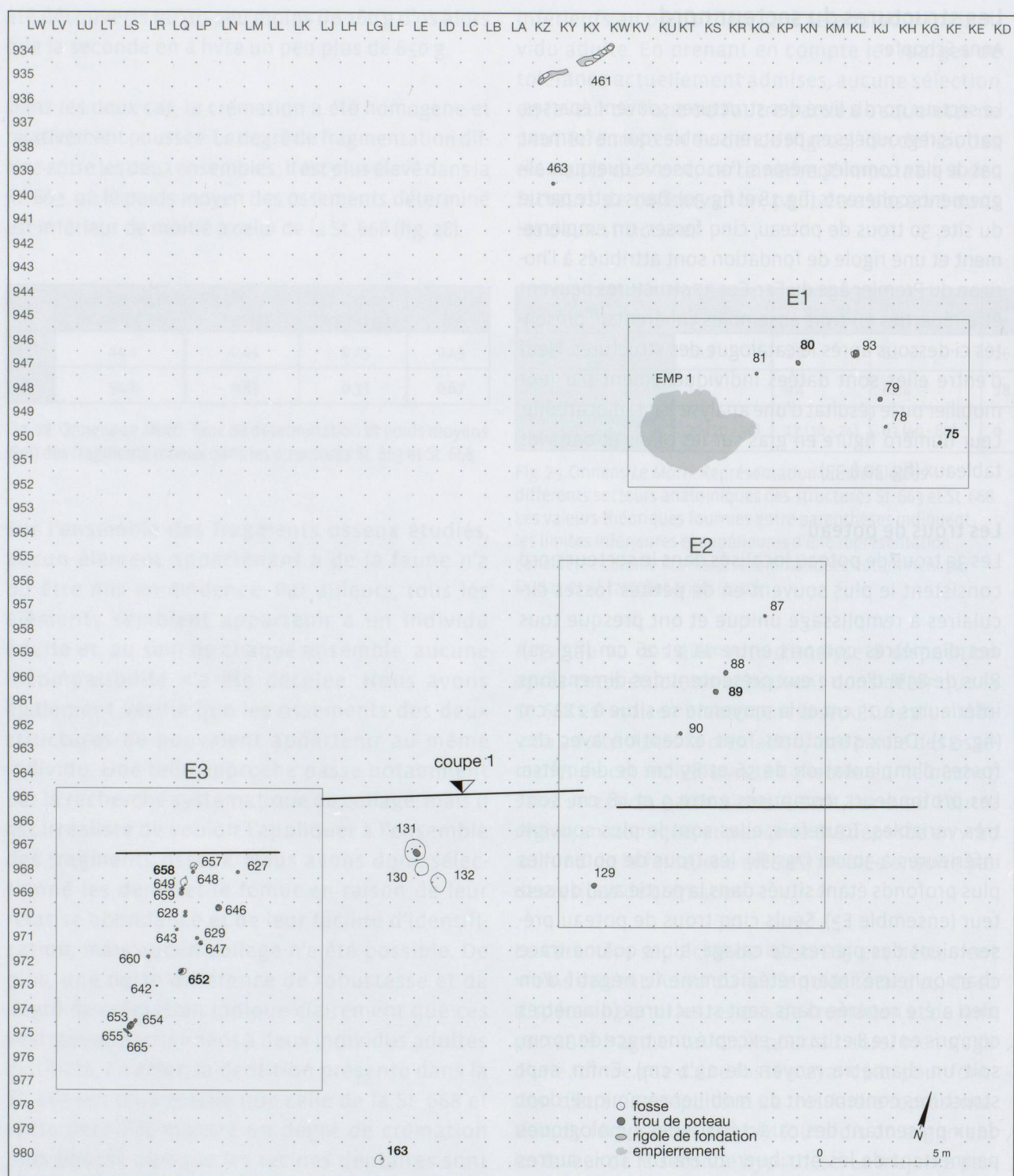
Fig. 30. Onnens-Le Motti. Plan général des structures du secteur nord avec (a) et sans (b) indication du numéro des structures et des ensembles.
