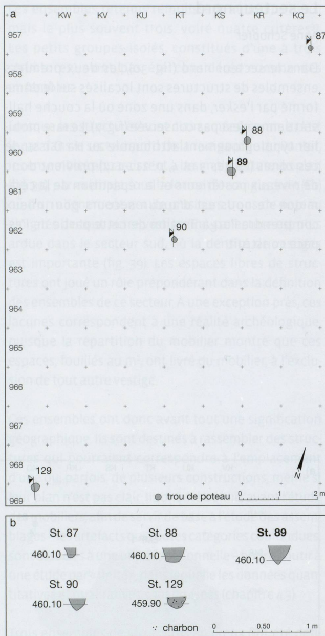
Fig. 75. Onnens-Le Motti. Plan de l'ensemble E2 (a) et relevé des coupes (b). Le numéro des structures datées individuellement figure en gras.
