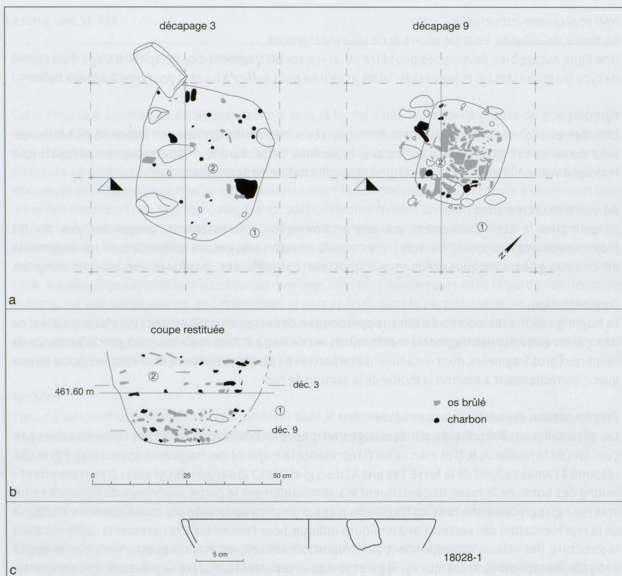
Fig. 24. Onnens-Le Motti. St. 668: plans (a), coupe restituée (b) et mobilier découvert en périphérie de la structure (c). Les couches 1 et 2 sont décrites dans le texte de présentation de la structure.
