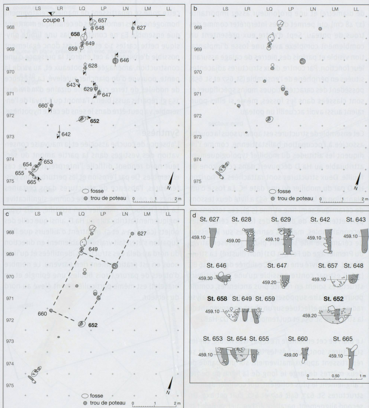
Fig. 76. Onnens-Le Motti. Plans de l'ensemble E3 avec (a) et sans (b) indication du numéro des structures; proposition de restitution (c) et relevés des coupes (d). Le numéro des structures datées individuellement figure en gras.
