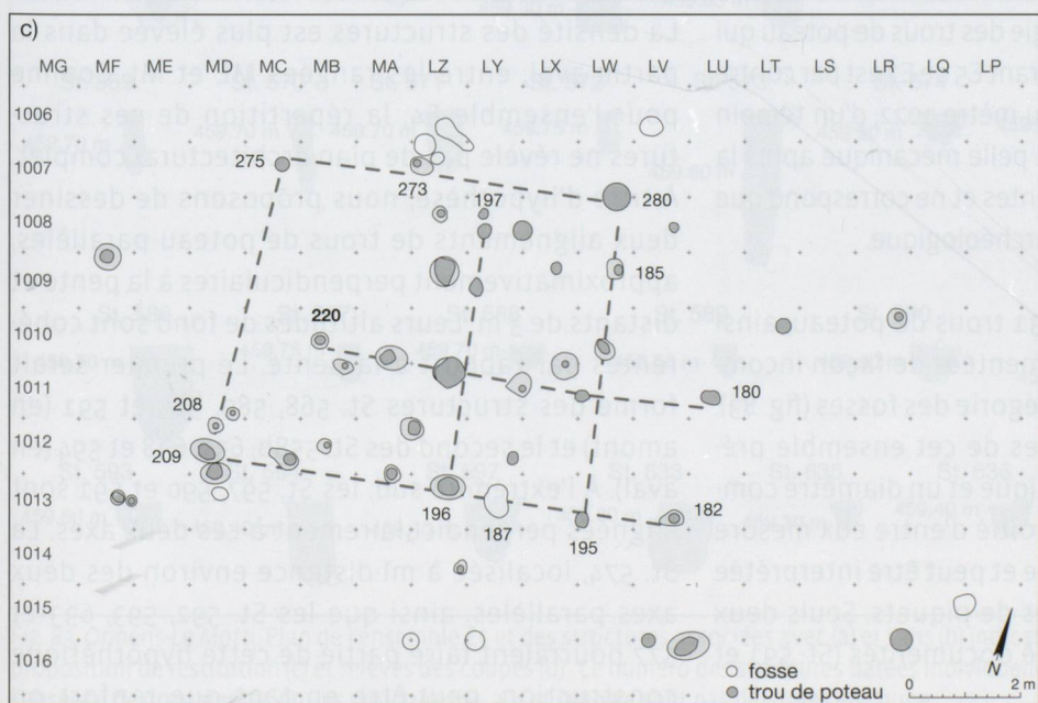
CI-CONTRE ET PAGE SUIVANTE Fig. 82. Onnens-Le Motti. Plans de l'ensemble E4 et des structures associées avec (a) et sans (b) indication du numéro des structures; proposition de restitution (c) et relevés des coupes (d). Le numéro des structures datées individuellement figure en gras. La coupe et le mobilier de la structure St. 187 sont présentés fig. 44.
