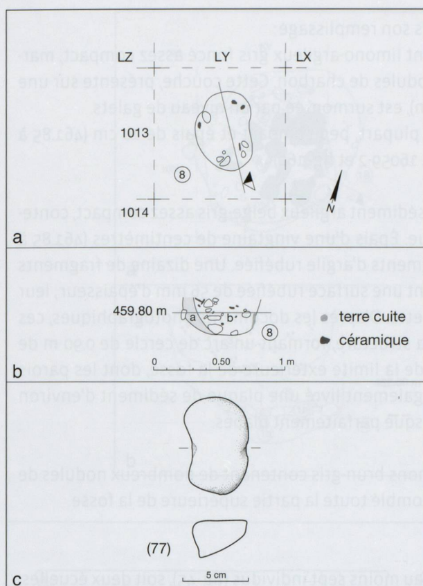
Fig. 44. Onnens-Le Motti. Plan (a), coupe (b) et mobilier de la fosse St. 187 (c). La couche 8 renvoie à la coupe de référence présentée au chapitre 2.2, p. 31.
