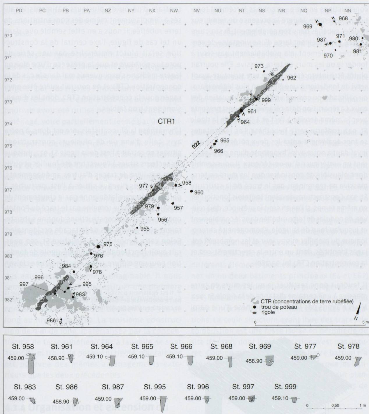
Fig. 87. Onnens-Le Motti. Plan des structures situées dans la moitié sud du secteur « rive droite » et relevé d'une partie des coupes des trous de poteau. Le numéro des structures datées individuellement figure en gras.
