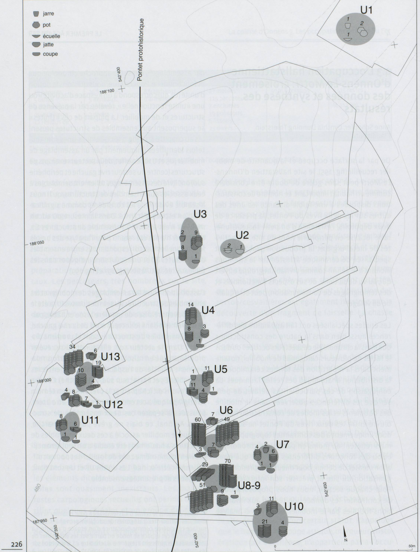
Fig. 196. Onnens-Le Motti. Localisation des 13 espaces d'activité identifiés pour l'occupation du Ha D et représentation graphique des ensembles céramiques associés. Les vases issus de contextes non stratifiés (U1 et U2) sont représentés en gris clair.
