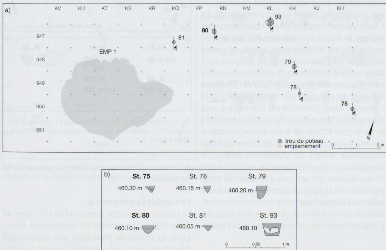
Fig. 74. Onnens-Le Motti. Plan de l'ensemble E1 (a) et relevé des coupes (b). Le numéro des structures datées individuellement figure en gras.
