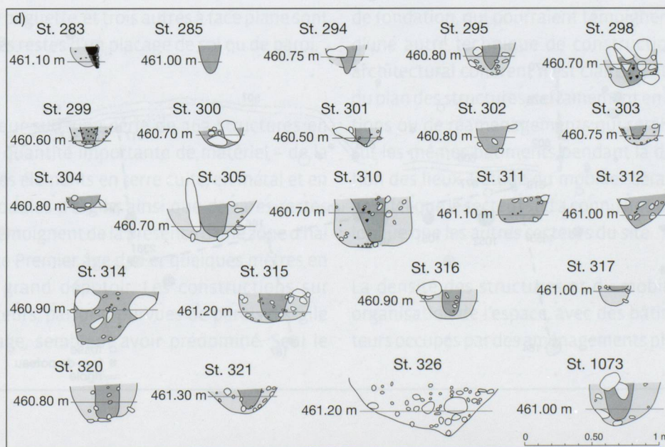
Fig. 84. Onnens-Le Motti. Plan de l'ensemble E6 et des structures associées avec (a) et sans (b) indication du numéro des structures; proposition de restitution (c) et relevés des coupes (d).
