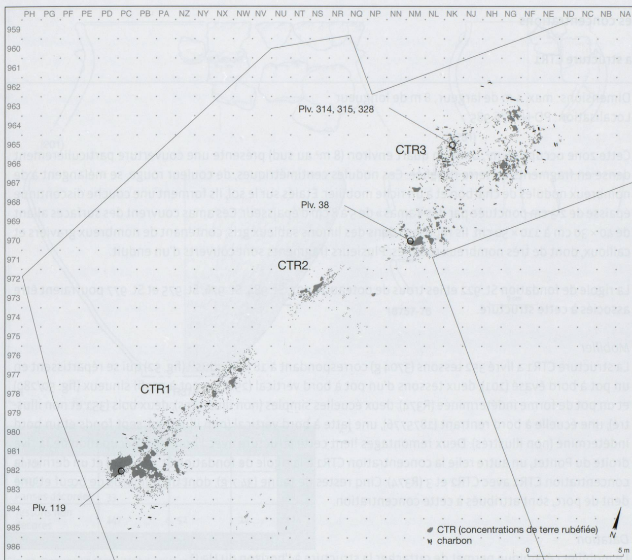
Fig. 51. Onnens-Le Motti. Localisation des fragments et des concentrations de terre rubéfiée sur la rive droite du Pontet. Les numéros (plv.) renvoient aux prélèvements de terre rubéfiée effectués sur le terrain (ci-dessous et annexe 3, fig. 245).
