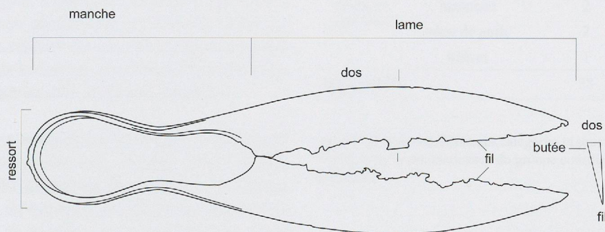
Fig. 54 Nomenclature des principaux éléments d'une paire de forces.
