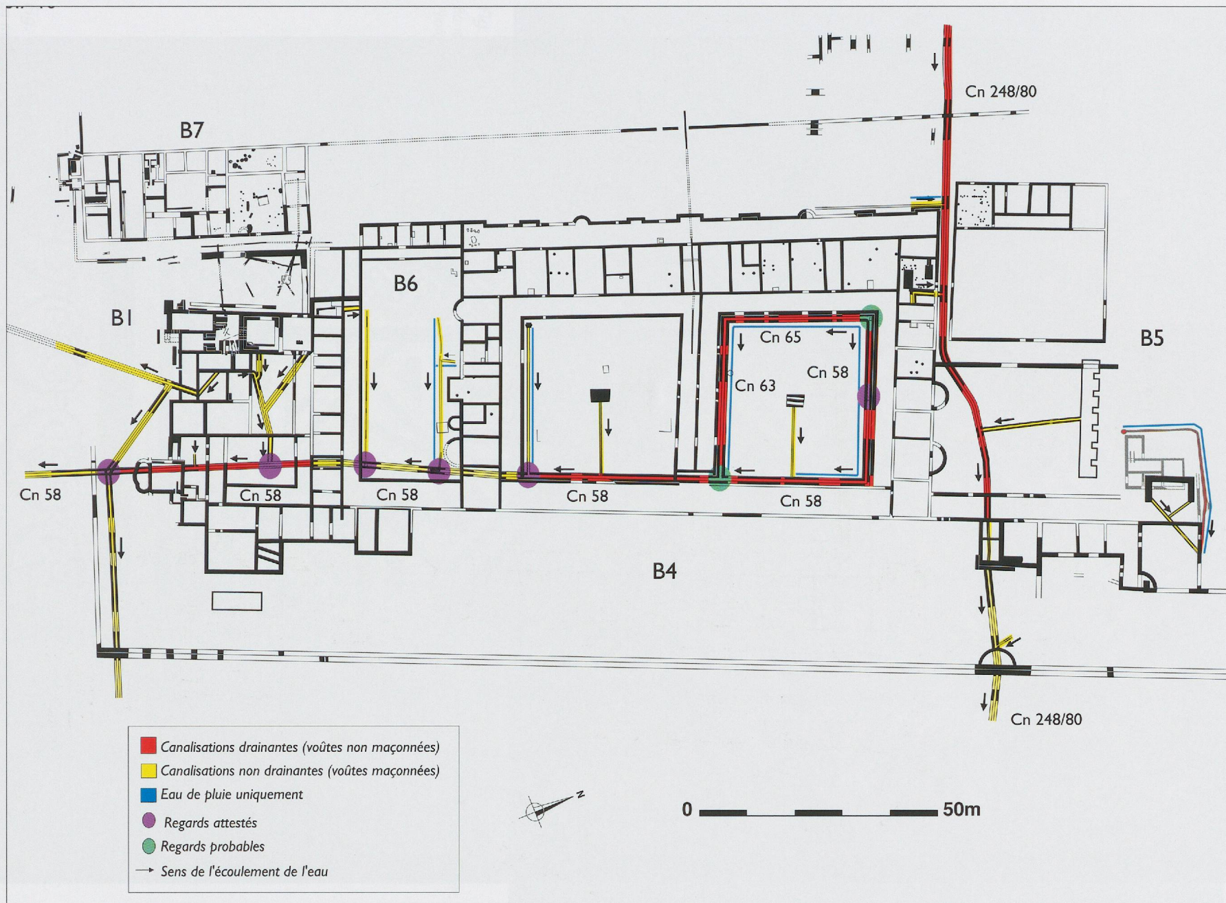
Plan de la pars urbana avec mise en évidence des deux réseaux d'évacuation: la partie nord est drainée par le collecteur Cn 248/80, entre les bâtiments B4 et B5, la partie centrale et le sud par le collecteur Cn 58/63/65. Les couvertures voûtées (types P et PTC) des canalisations sont par endroits drainantes (dépourvues de mortier), pour permettre un meilleur assainissement des sols (d'après Tissot 2001, vol. 1, p. 58, et REMONDIN 1996, p. 101-102).
