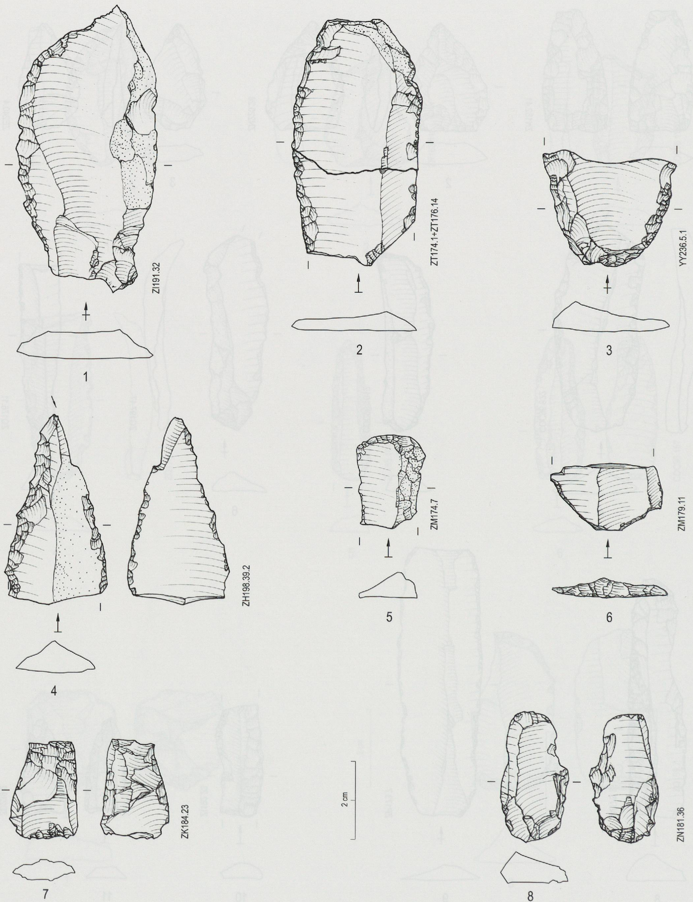
Planche 113. Ensemble E5. 1 et 3 Éclats retouchés. 2 lame retouchée. 4 Burin. 5 Grattoir court simple. 6 Éclat à enlèvements irréguliers. 7 et 8 Pièces esquillées (éch. 1 : 1).
