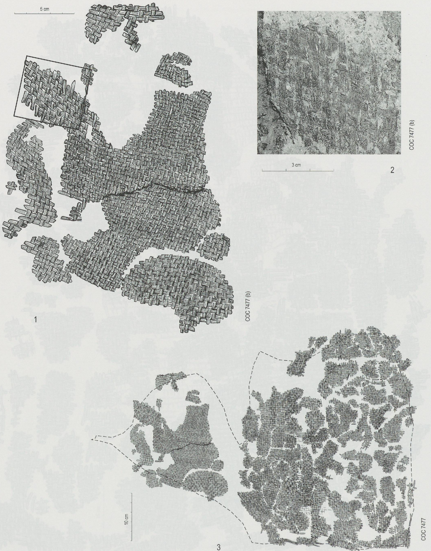
Planche 63. Ensemble E2. Natte ou vannerie à brins entrelacés en armure toile. 1 Second fragment de l'objet COC7477 (éch. 1 : 2). 2 Détail (éch. 1 : 1). 3 Position relative des 2 fragments (éch. 1 : 5).
