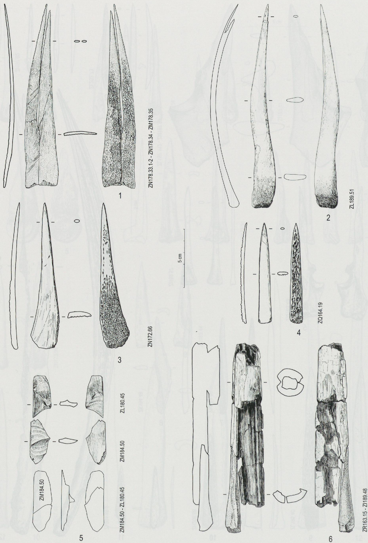
Planche 25. Ensemble E2. 1 Raccord entre deux pointes de peigne à carder type P2. Pointes de peigne à carder : 2 type P5 ; 3, 4 type P2 recyclées. 5 Remontage de deux fragments indéterminés. 6 Remontage d'un métapode de cerf, déchet de fabrication brûlé (éch. 1 : 2).
