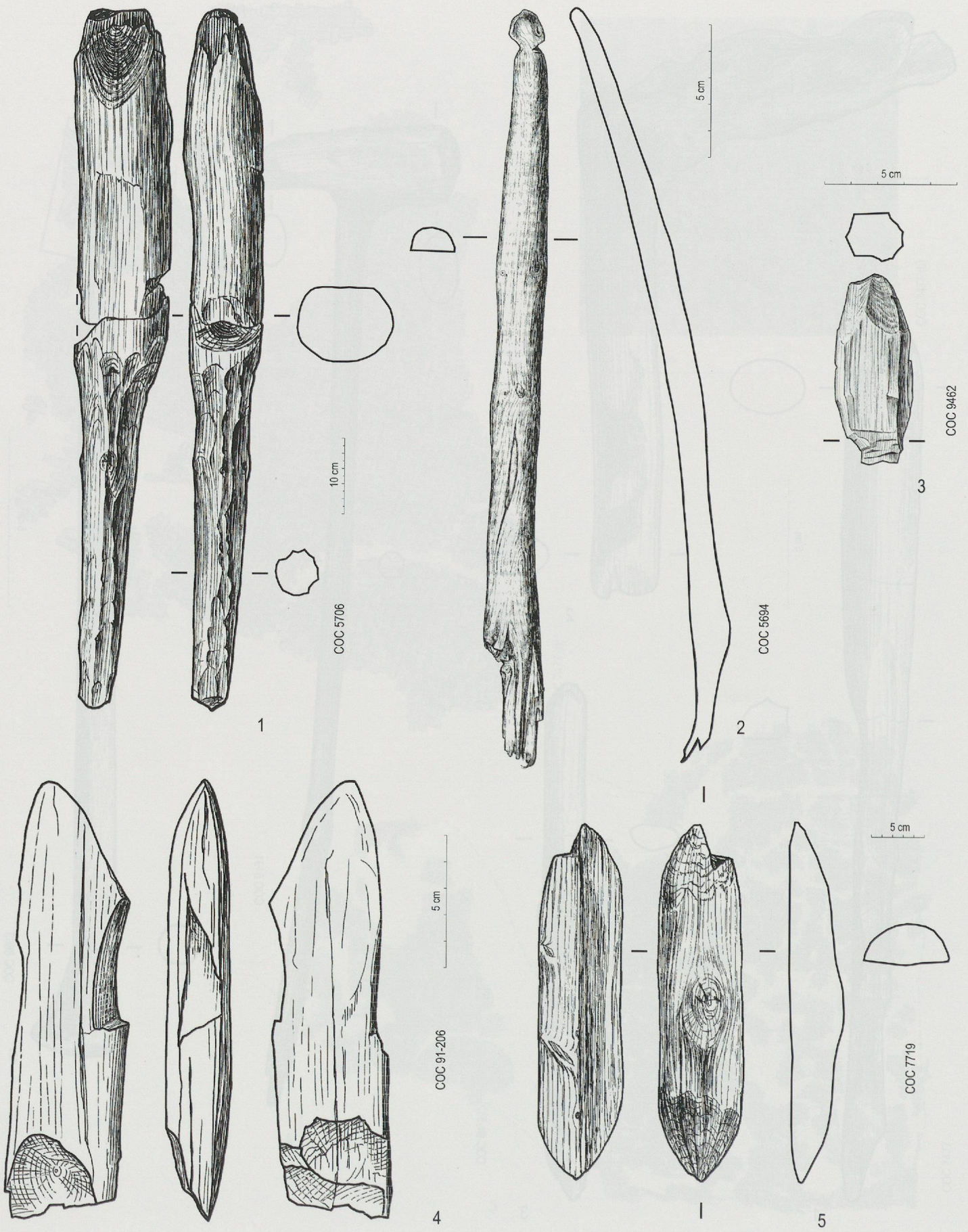
Planche 65. Ensemble E2. 1 Masse en chêne (éch. 1 : 7). 2 Fragment d'arc en if. 3 Chute de taille ou tampon en érable. 4 Flotteur en chêne (éch. 1 : 2). 5 Double pointe en chêne (éch. 1 : 5).
