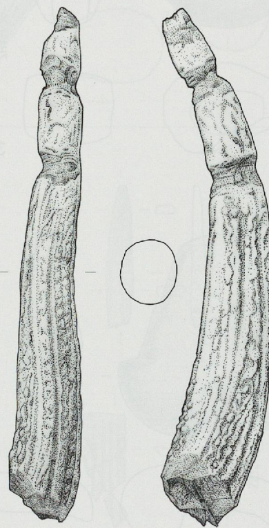
Planche 14. Ensemble E4. 1, 2 Outils à perforation transversale. Ensemble E5. 3 Outil à perforation transversale. 4 Andouillier central avec ébauche de débitage, chute de type 5b (éch. 1 : 2).
