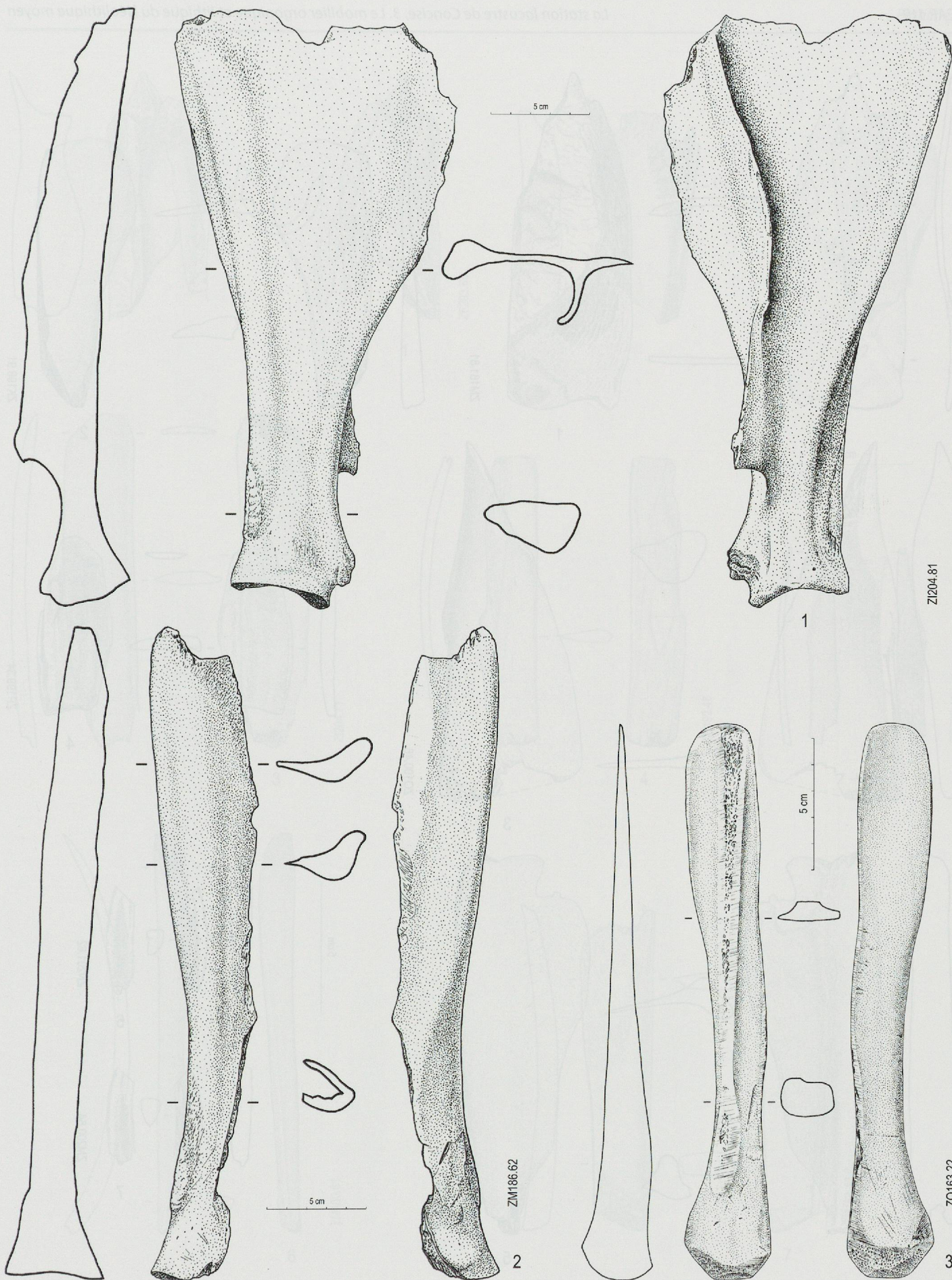
Planche 30. Ensemble E2. 1 Omoplate avec traces de manipulation, pelle ? 2 Scapulas de bœuf, ébauche de fabrication d'un biseau. 3 Pièce à tranchant transversal type biseau (éch. 1 : 2).
