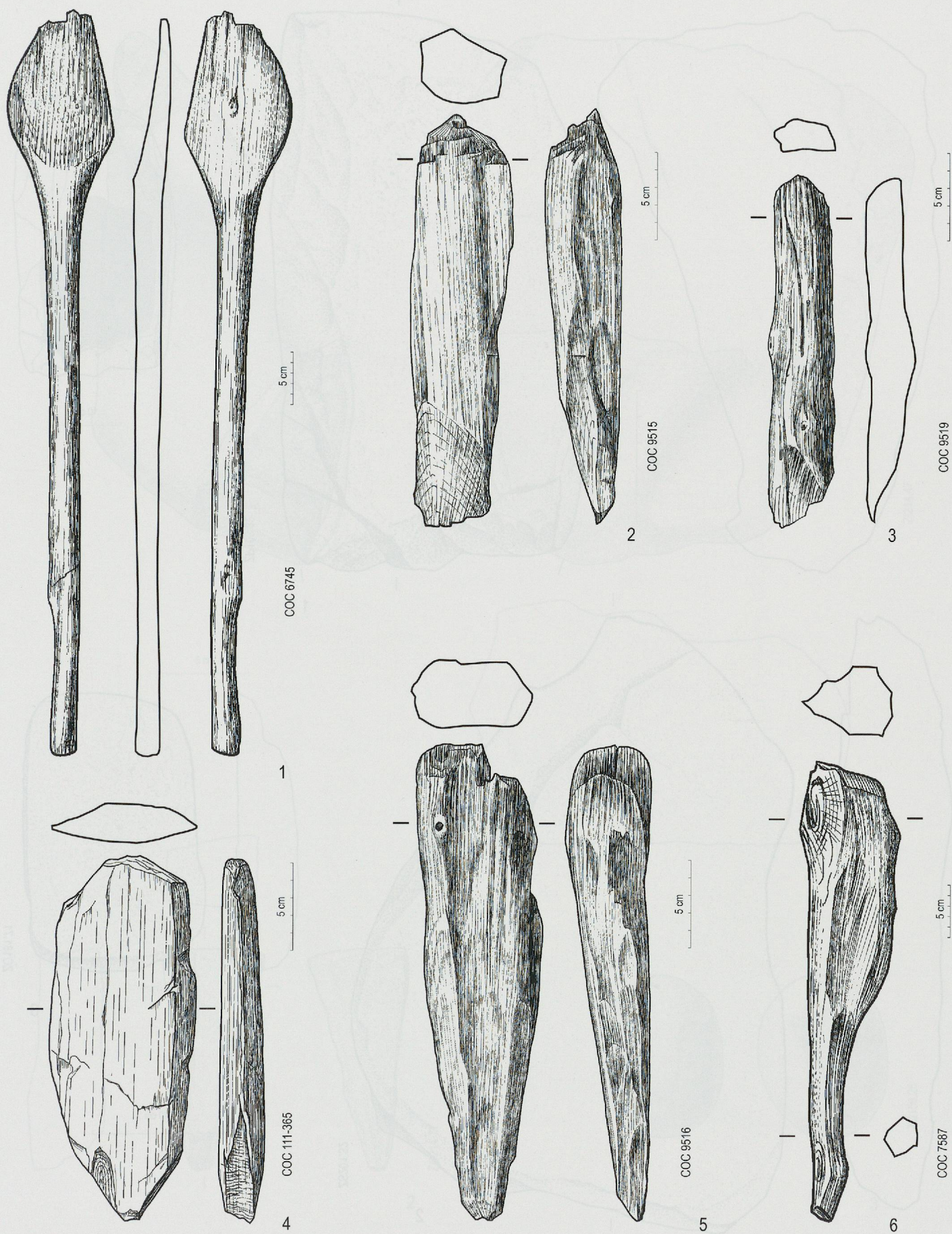
Planche 80. Ensemble E5. 1 Palette ou pelle en érable (éch. 1 : 5). 2 Coin à fendre. 3, 5 Coins. 4 Déchet de taille (éch. 1 : 3). 6 Masse en chêne (éch. 1 : 5).
