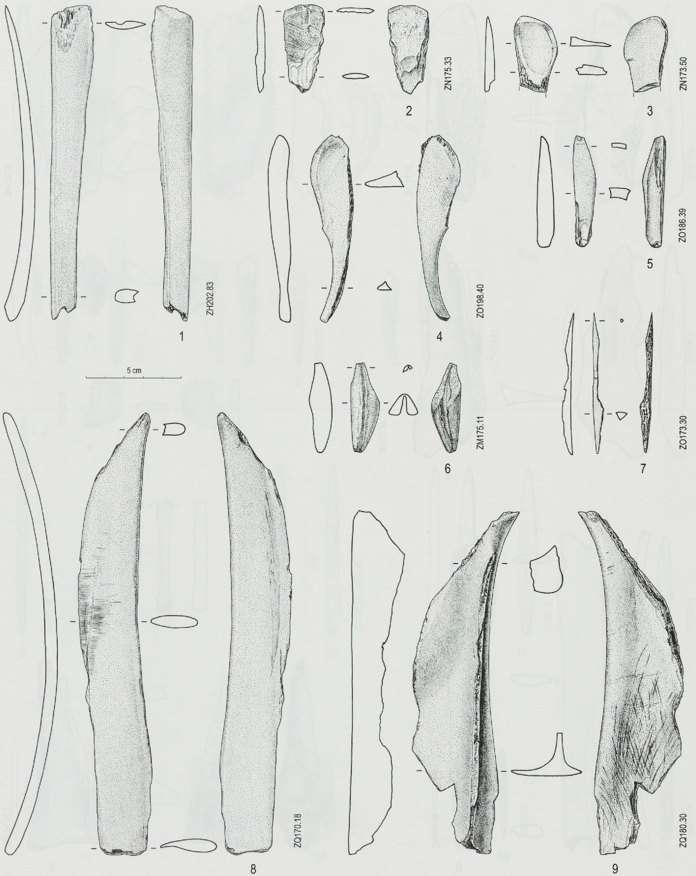
Planche 38. Ensemble E3. Biseaux : 1 type B5 ; 2 type B3 ; 3 type indéterminé ; 5 type B1. Chanfreins : 4 sur coxal de bœuf ; 6 sur ivoire. 7 Fragment d'outil sur côte. 8 Lissoir sur côte. 9 Scapula de bœuf avec incisions et profond lustré (éch. 1 : 2).
