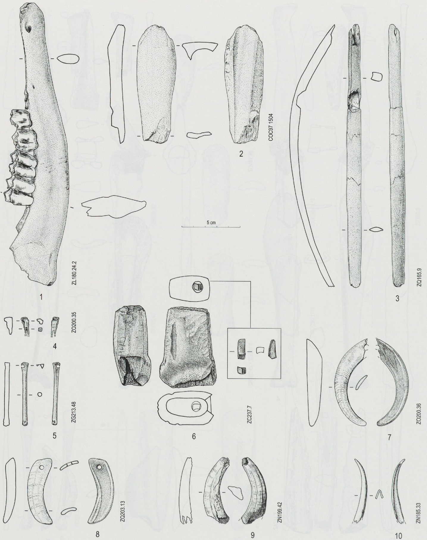
Planche 45. Ensemble E4. 1 Élément à impressions type retouchoir sur mandibule de cerf. 2 Pièce intermédiaire. 3 Élément à impressions type lisseur. Pendeloques : 4, 5 sur os ; 7, 8 sur ivoire. 6 Coin de calage dans une gaine en bois de cerf. 9 Compresseur sur ivoire. 10 Fragment indéterminé d'une canine inférieure de suidé (éch. 1 : 2).
