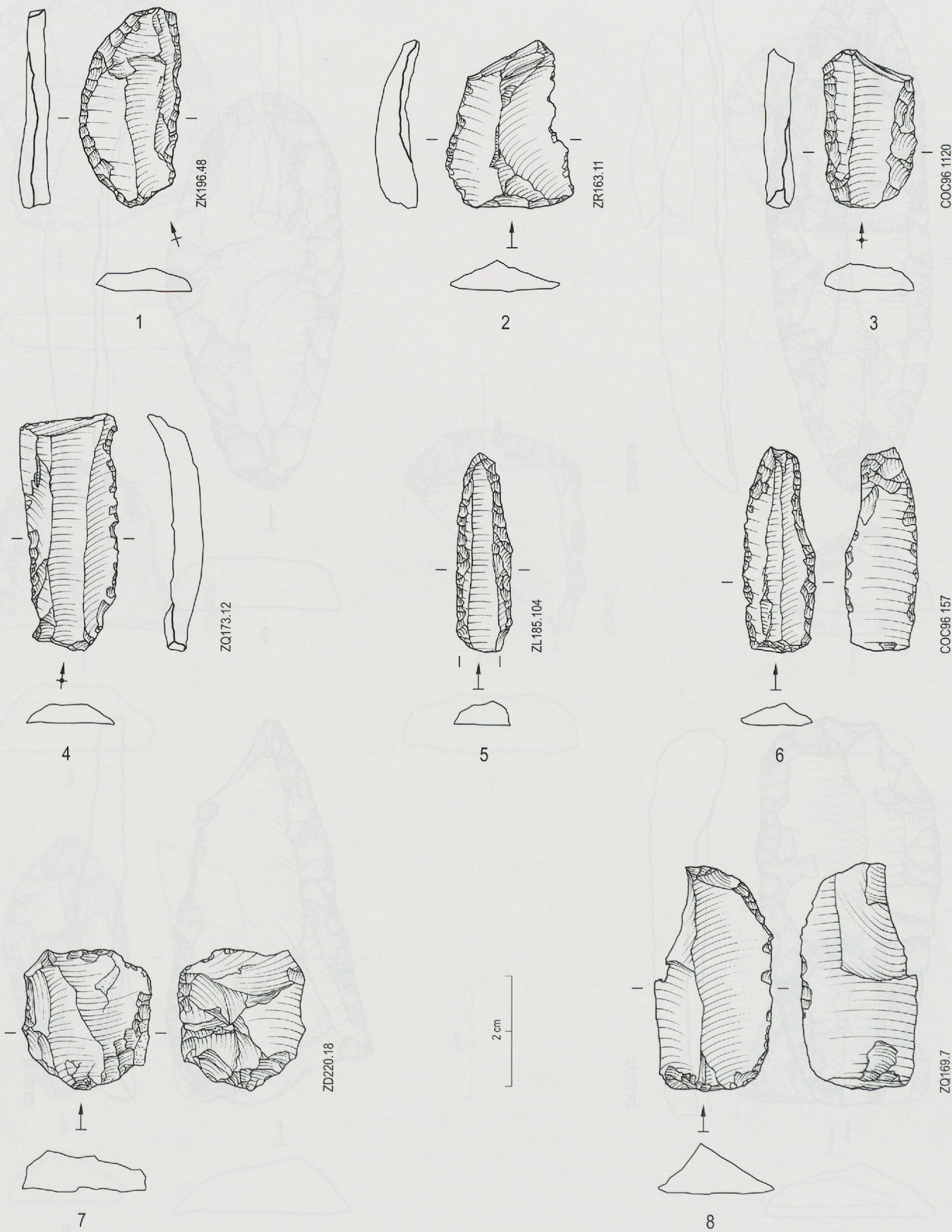
Planche 111. Ensemble E4. 1 Éclat retouché. 2 Éclat à enlèvements irréguliers. 3 Lamelle retouchée. 4 Lamelle à enlèvements irréguliers. 5 et 6 Lamelles retouchées. 7 et 8 Pièces esquillées (éch. 1 : 1).
