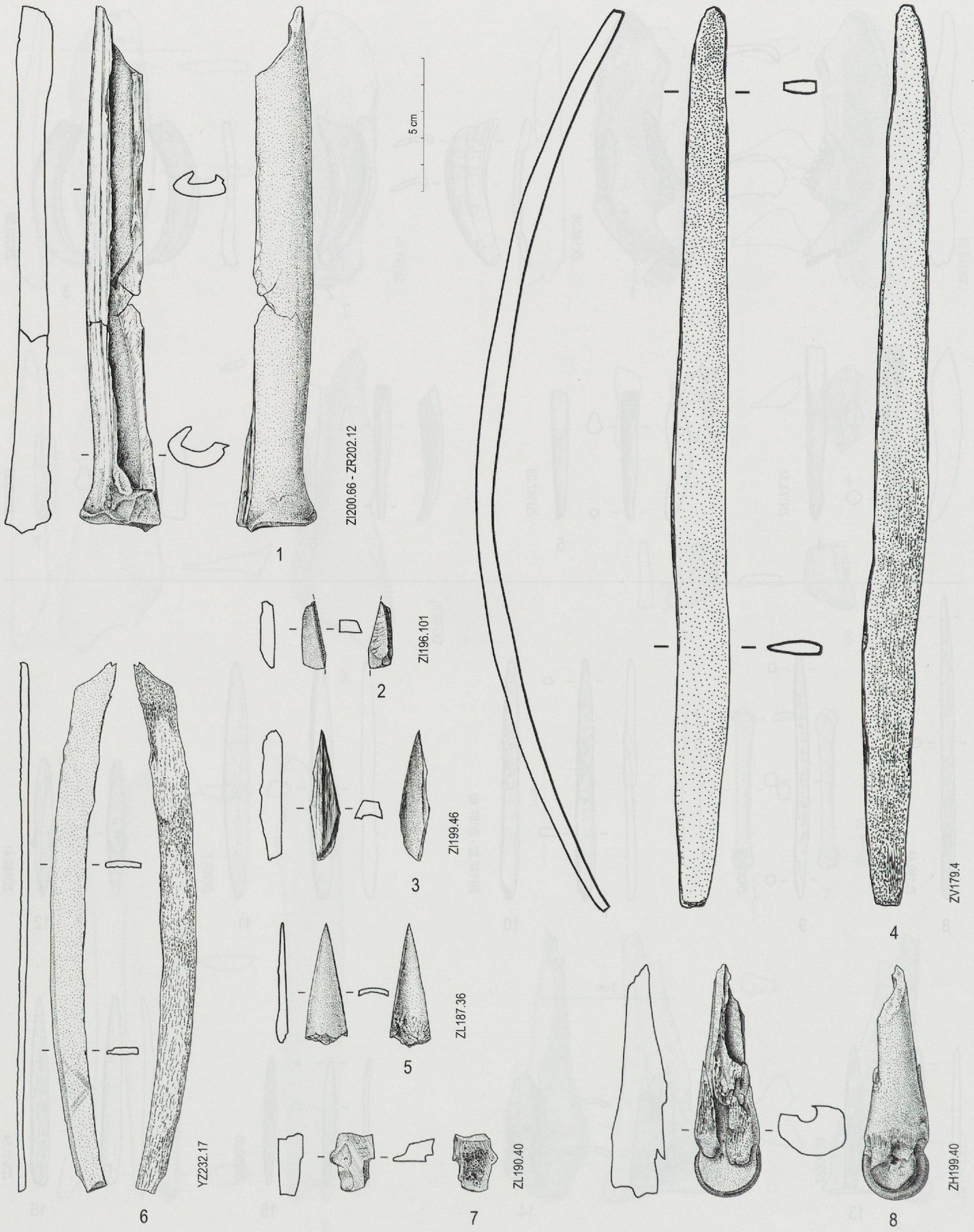
Planche 41. Ensemble E4. Déchets de fabrication sur os (éch. 1 : 2).
