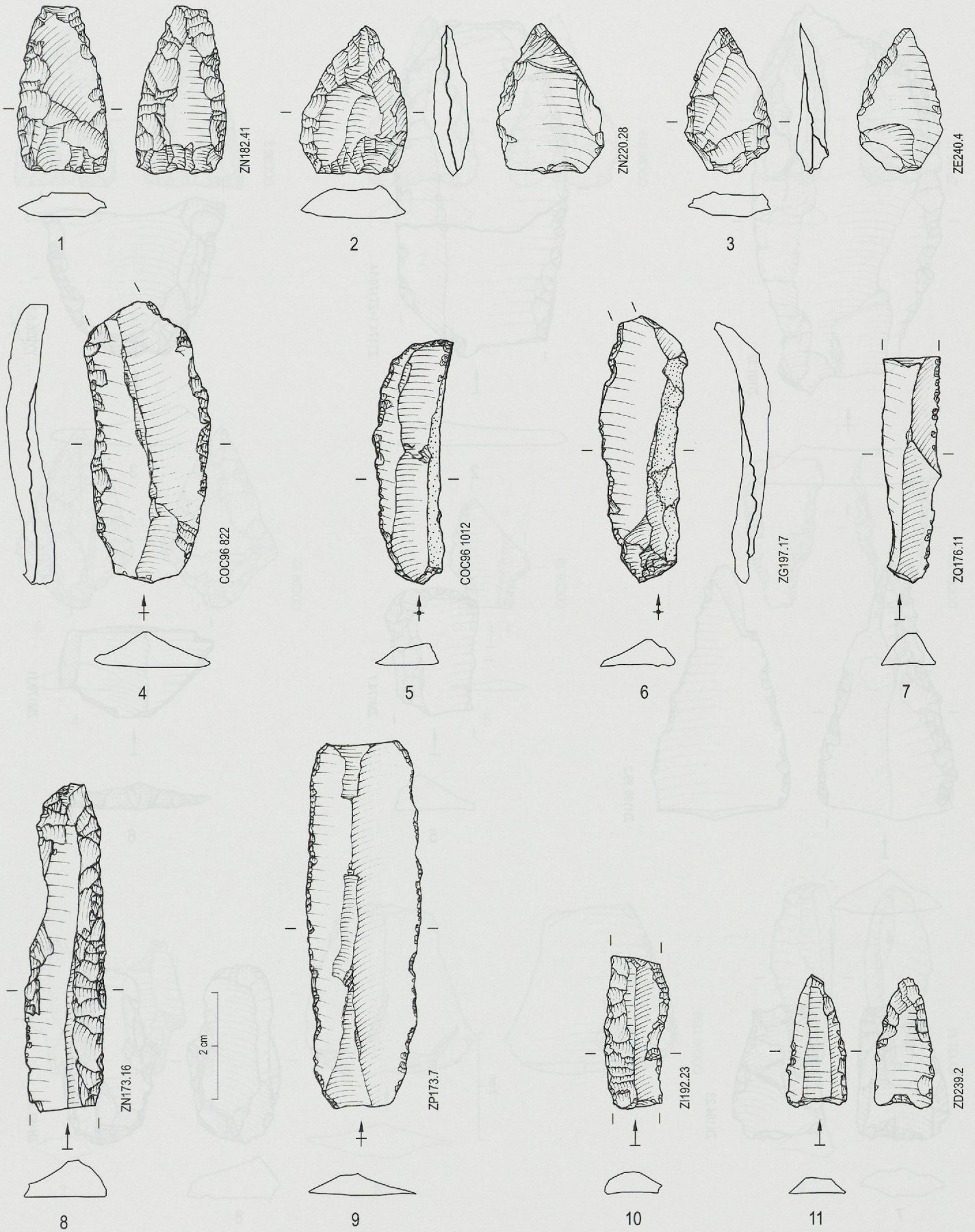
Planche 112. Ensemble E5. 1 à 3 Pointes de flèche triangulaires. 4 à 6, 8 à 11 Lames et lamelles retouchées. 7 Lamelle microdentículée (éch. 1 : 1).
