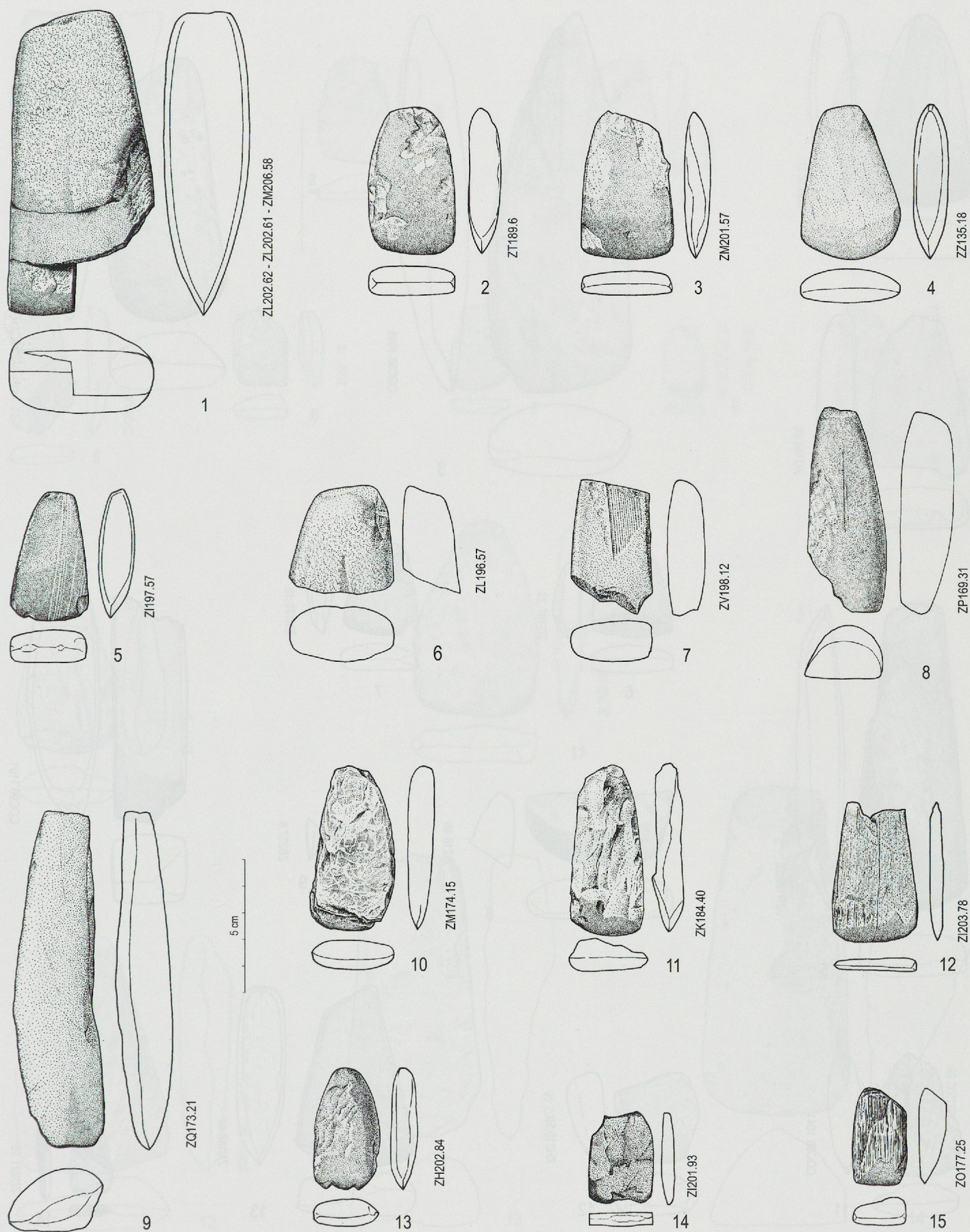
Planche 122. Ensemble E3. 1 Hache de type 1. 2 à 4 Haches de type 3. 5 Hache de type 5 en pélite-quartz. 6 à 8 Fragments de haches de type indéterminé. 9 Ebauche de hache. 10 à 15 Tranchets (éch. 1 : 2).
