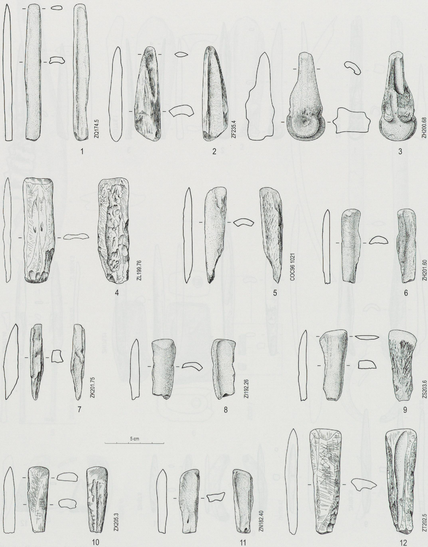
Planche 47. Ensemble E5. Biseaux : 1, 2 type B1 ; 3 type B2 ; 4-11 type B3 ; 12 type B4 (éch. 1 : 2).
