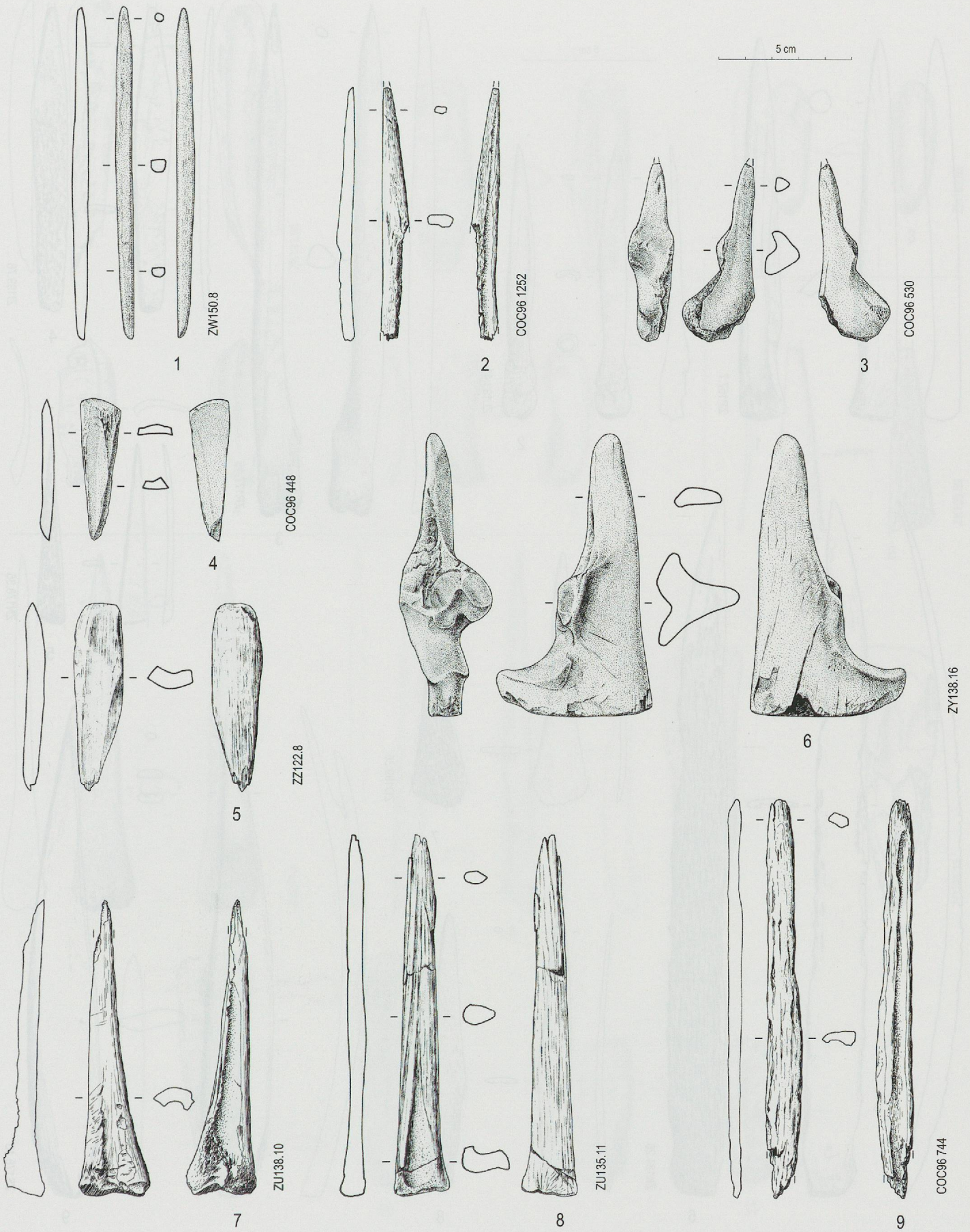
Planche 50. Ensemble E6. 1 Pointe de projectile type P3A. 2 Pointe type indéterminé. 3 Poinçon type P4. Biseaux : 4, 5 type B3 ; 6 type B5. 7, 8 Déchets de fabrication sur métapodes. 9 Objet fini indéterminé (éch. 1 : 2).
