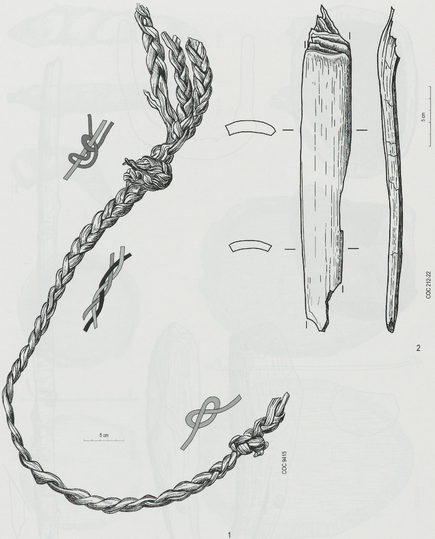
Planche 54. Ensemble E1. 1 Cordage formé de deux tresses à trois brins assemblées par un nœud (éch. 1 : 3). 2 Fragment d'un arc en if ? (éch. 1 : 2).
