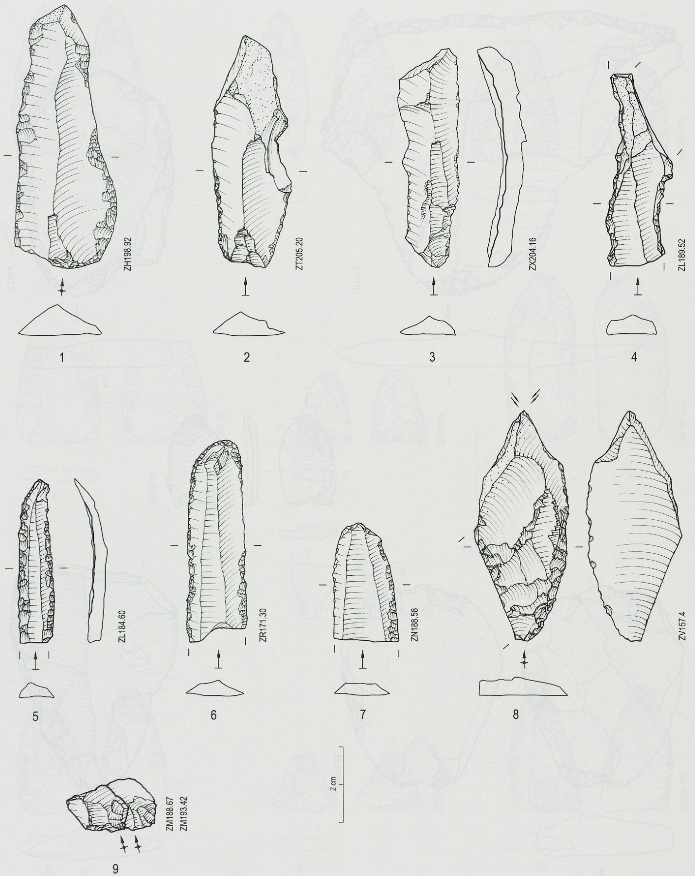
Planche 106. Ensemble E2. 1 à 3 Lames à enlèvements irréguliers. 4 à 7 Lames et lamelles à retouches latérales. 8 Burin dièdre. 9 Remontage de deux éclats de retouche (éch. 1 : 1).
