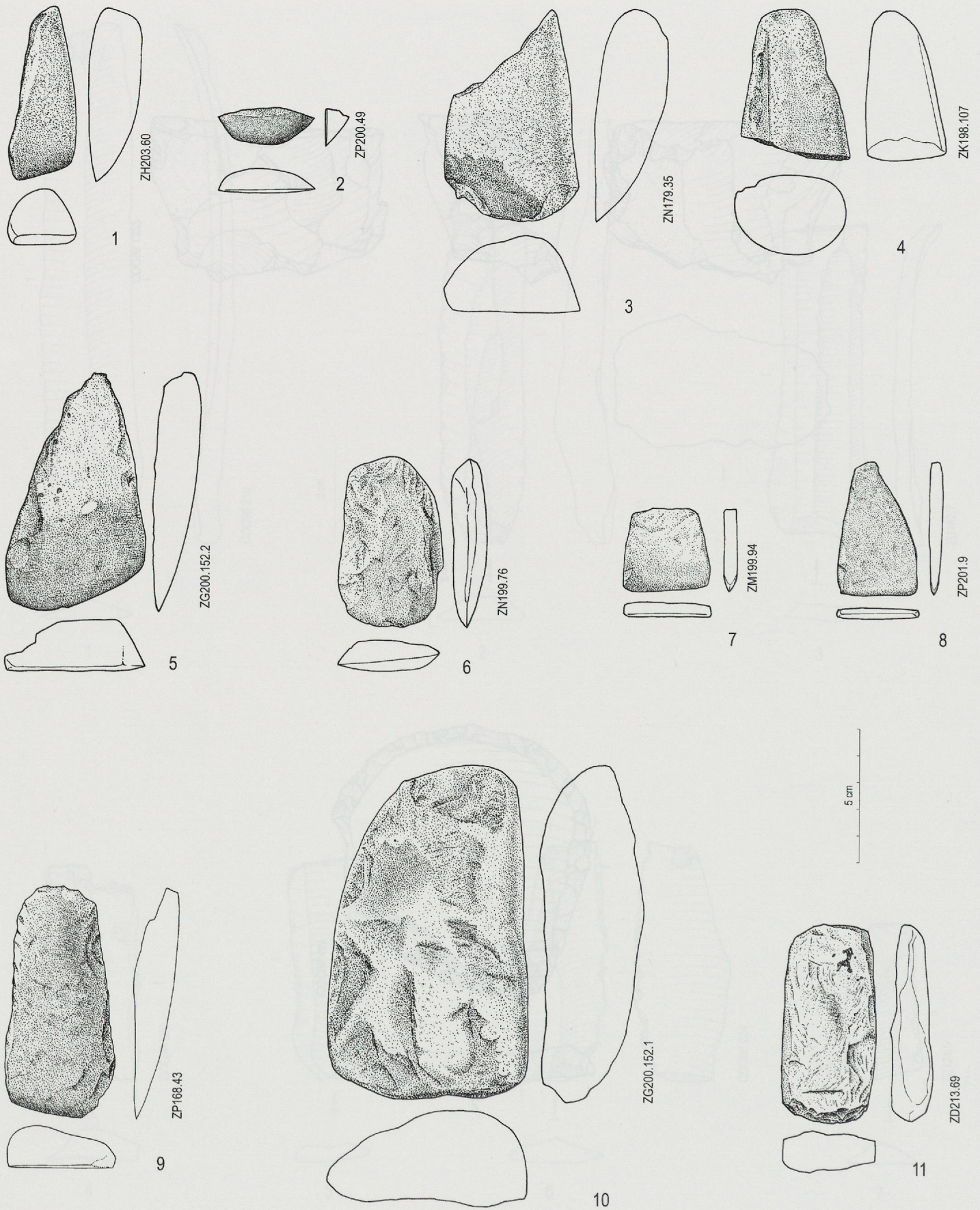
Planche 117. Ensemble E1. 1 Hache de type 1. 2 à 4 Fragments de haches de type indéterminé. 5 à 9 Tranchets. 10 et 11 Ebauches de haches de type indéterminé (éch. 1 : 2).
