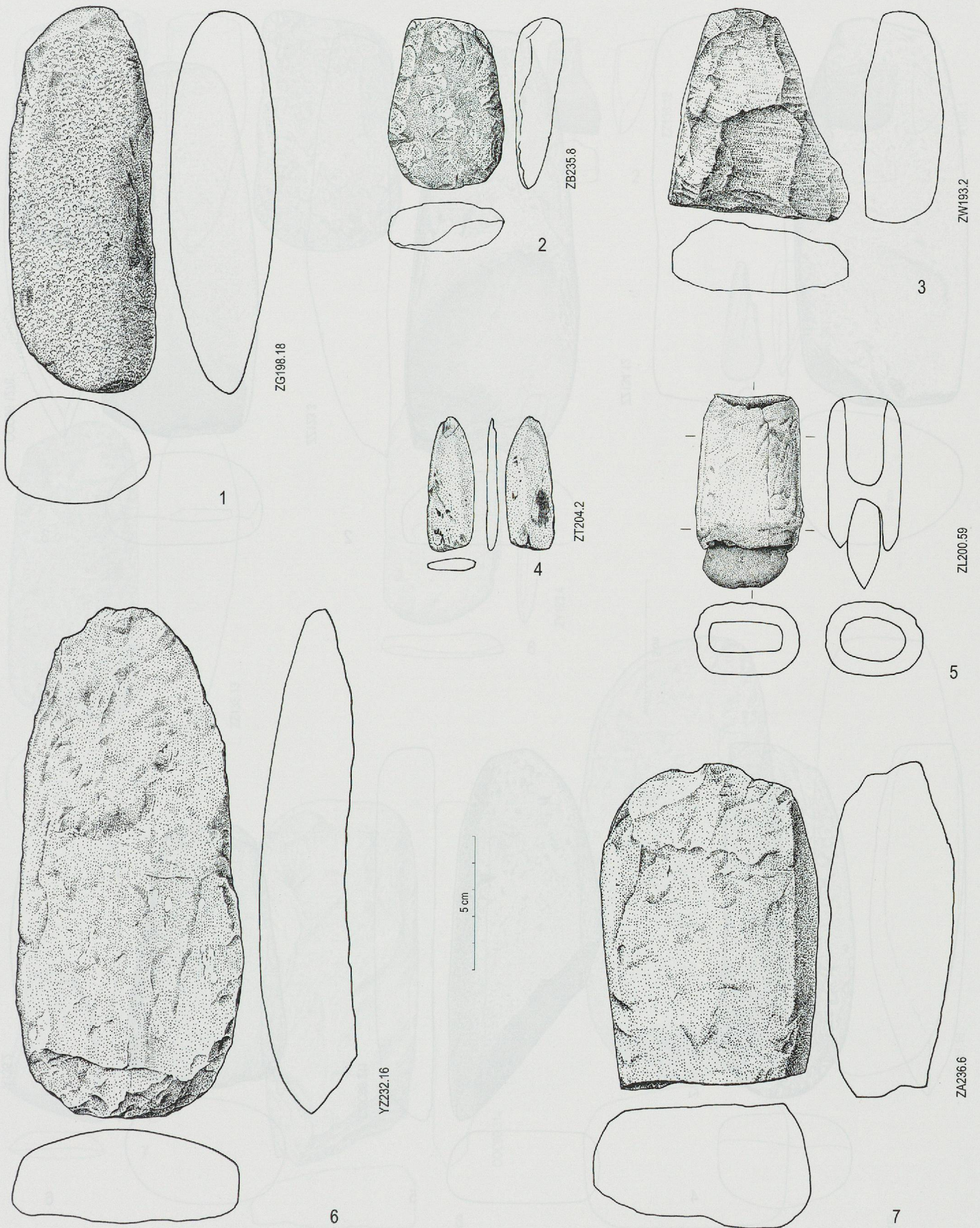
Planche 126. Ensemble E5. 1, 3, 6 et 7 Ebauches de haches de type indéterminé. 2 Ebauche de hache de type 4. 4 Pointe de flèche en néphrite. 5 Hache de type 2 dans sa gaine à double douille (éch. 1 : 2).
