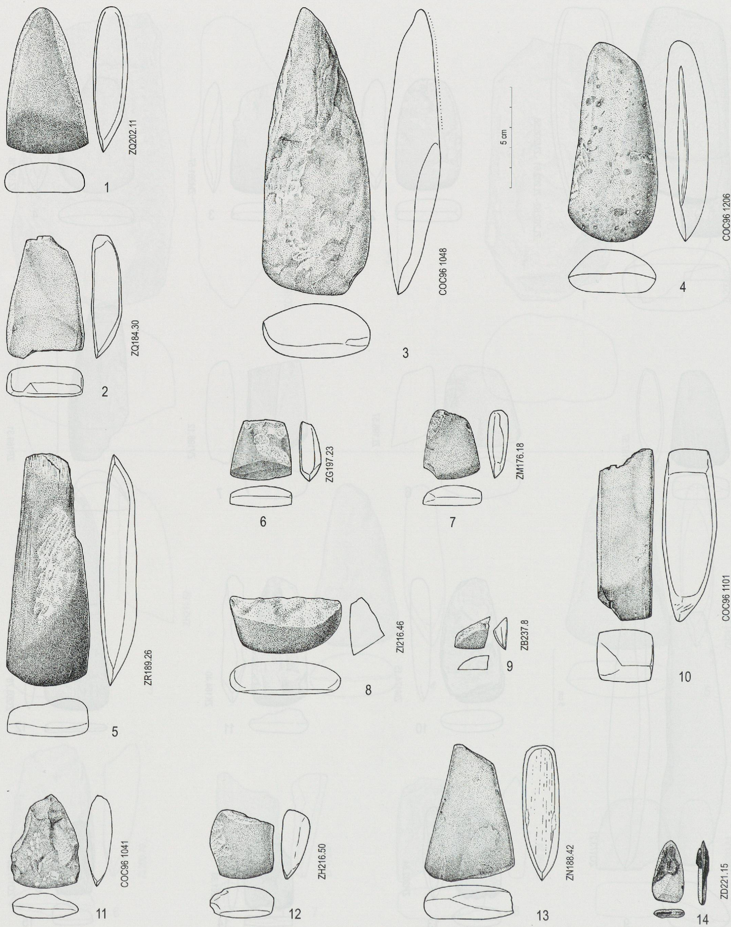
Planche 123. Ensemble E4. 1 et 2 Haches de type 2. 3 à 9 Haches de type 3. 10 Hache de type 5 en pépite-quartz. 11 Hache de type 4. 12 et 13. Bouchardes sur fragment de hache en jadéite. 14 Pointe de flèche en néphrite (éch. 1 : 2).
