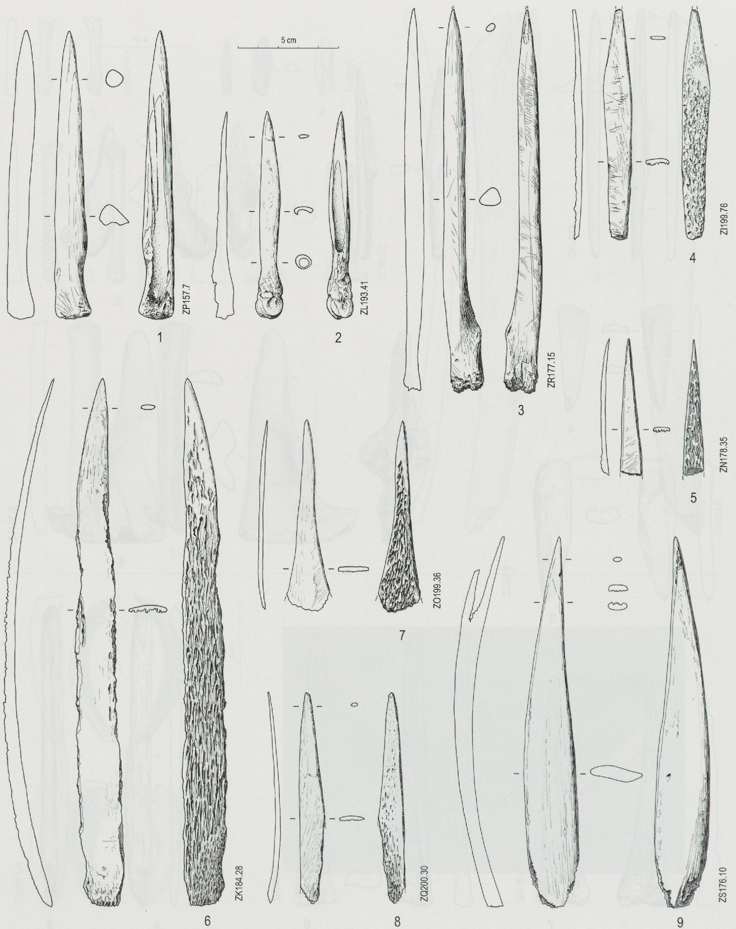
Planche 51. Lot « NM » : Néolithique moyen, mélange, matériel provenant des structures. Poinçons : 1, 2 type P1A ; 3 type P4. Pointes de peigne à carder : 4-8 type P2 ; 9 type P5 (éch. 1 : 2).
