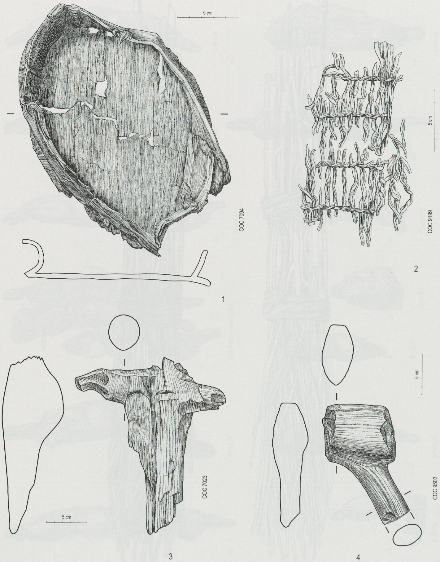
Planche 69. Ensemble E3. 1 Panier en écorce. 2 Etoffe cordée, variante A de la catégorie C de Vogt (1937) (éch. 1 : 2). 3 Tête de pioche ? en sapin. 4 Maillet en chêne (éch. 1 : 3).
