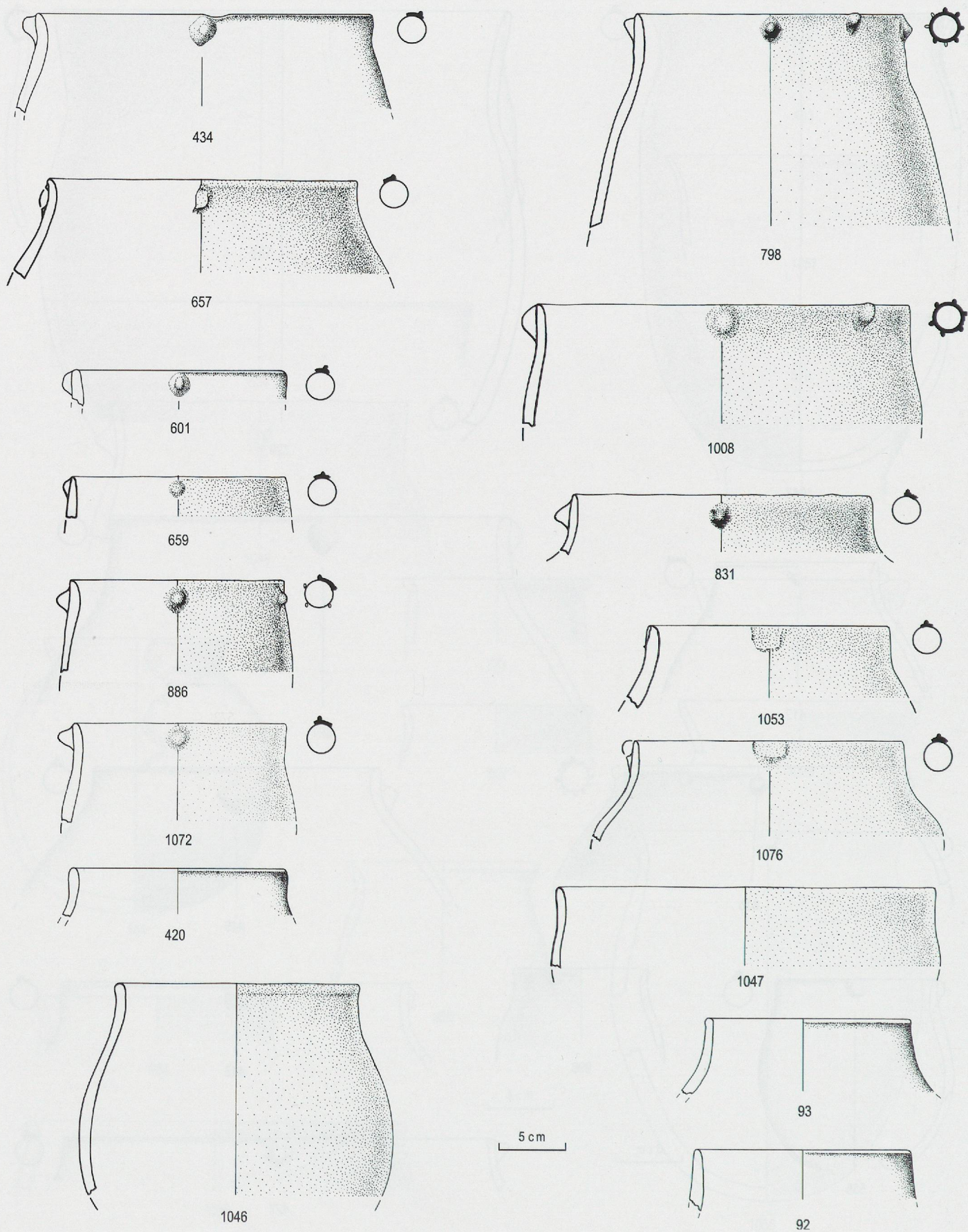
Planche 11. Ensemble E2. Jarres à bord vertical (type j20). Ech. 1 : 4.
