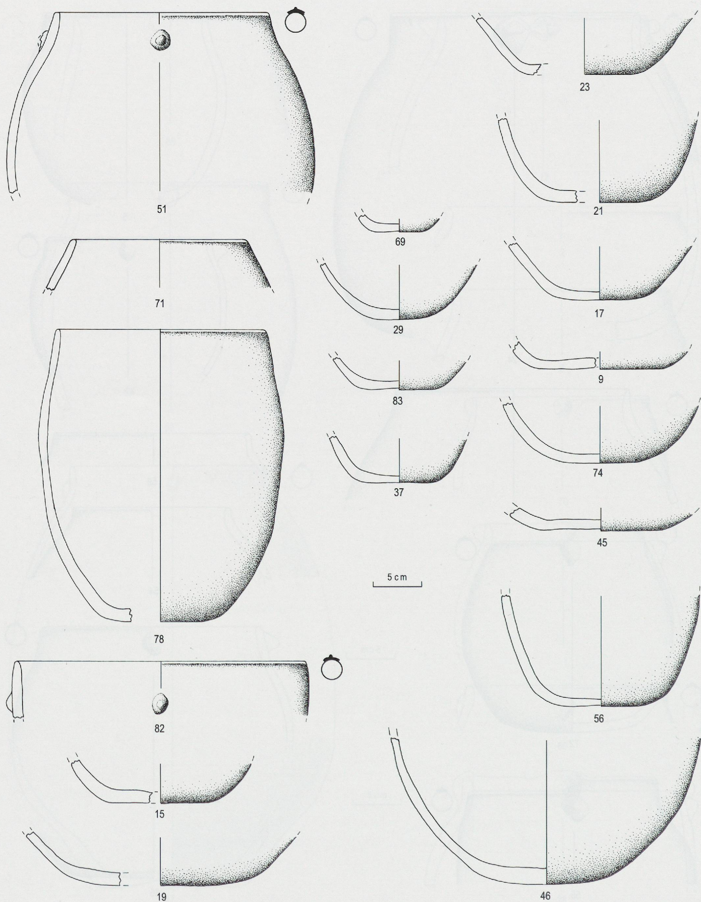
Planche 73. Ensemble E6. Jarres non segmentées à bord rentrant (type j30 : 51, 71, 78), en pot de fleur (type j22 : 82). Jarres indéterminées. Ech. 1 : 4.
