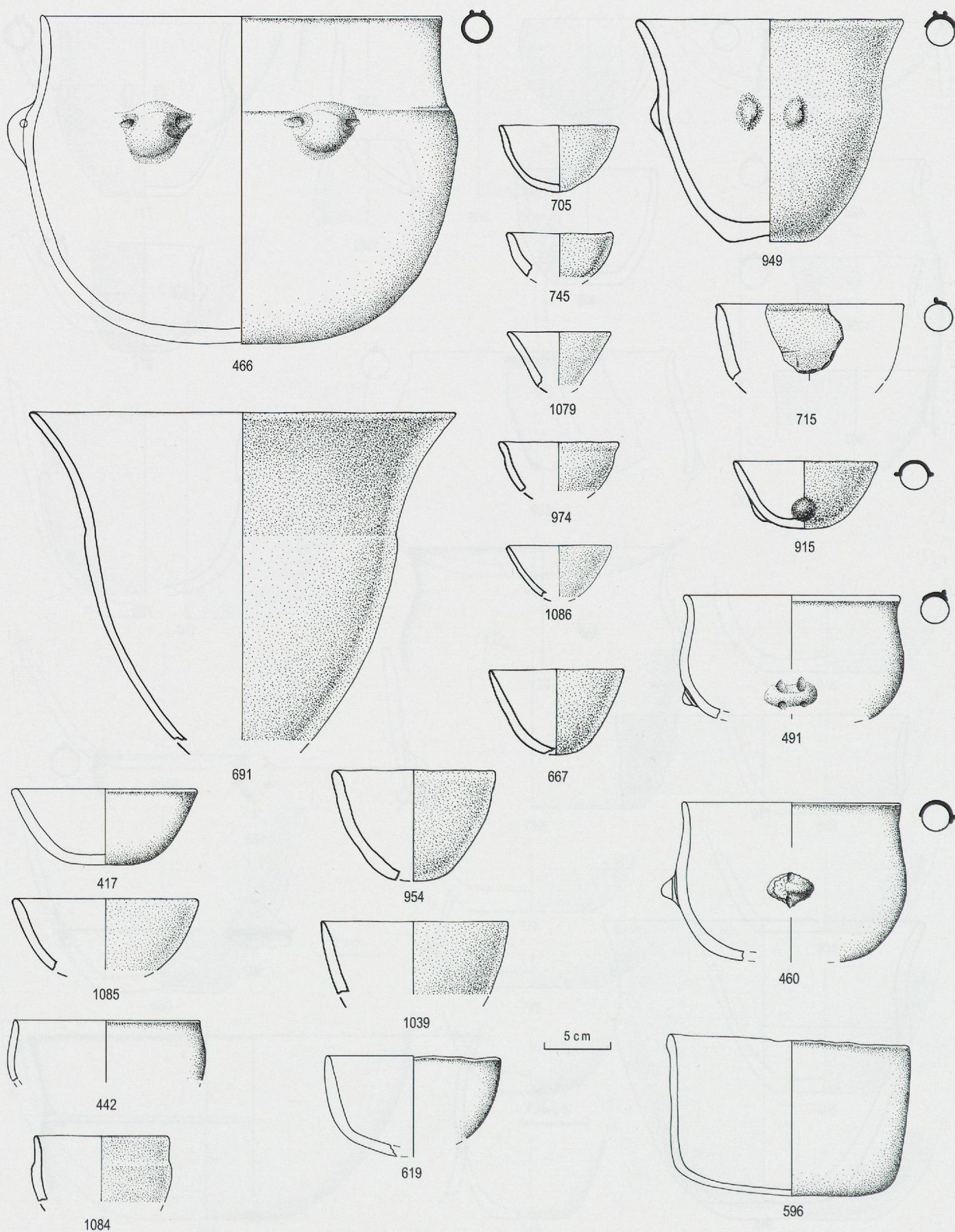
Planche 23. Ensemble E2. Marmites segmentées (type m40 et m50 : 466, 691, 949). Bols non segmentés (417, 442, 619, 667, 705, 715, 745, 915, 954, 974, 1039, 1079, 1085, 1086) ou segmentés (1084). Jattes à profil en S (type jj10 : 460, 491) ou à bord vertical (type jj22 : 596). Ech. 1 : 4.
