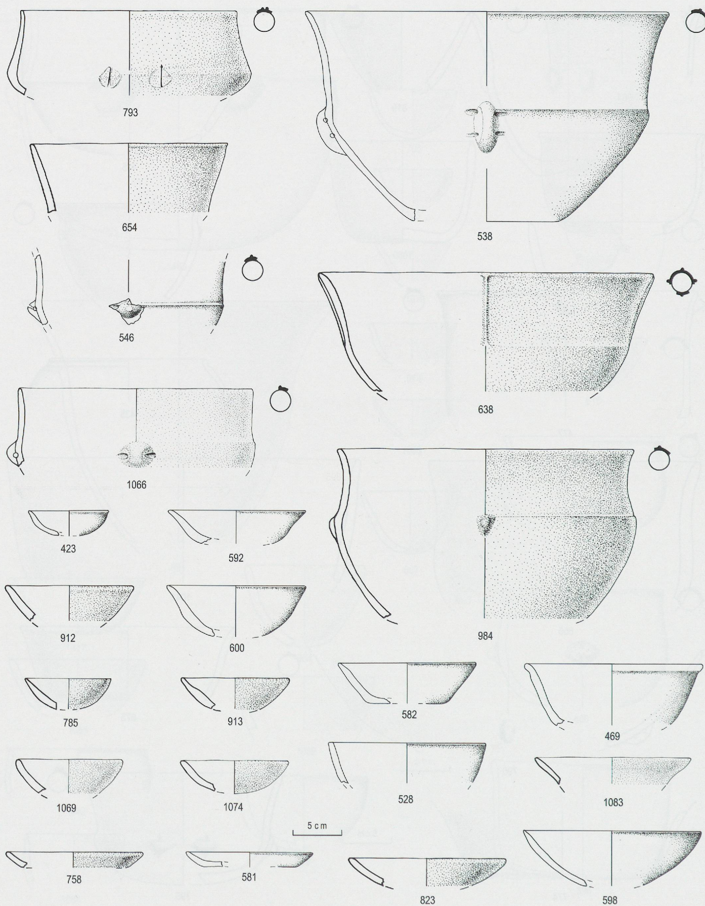
Planche 25. Ensemble E2. Grandes jattes à paroi rectiligne ouverte (type Jj11 : 654), à segmentation basse (type Jj52 : 793), à épaule et bord évasé (type Jj40 : 538, 546, 638, 984) ou vertical (type Jj50 : 1066). Coupes (423, 581, 582, 592, 600, 758, 785, 912, 913, 1069, 1074). Ecuelles (469, 528, 598, 823, 1083). Ech. 1 : 4.
