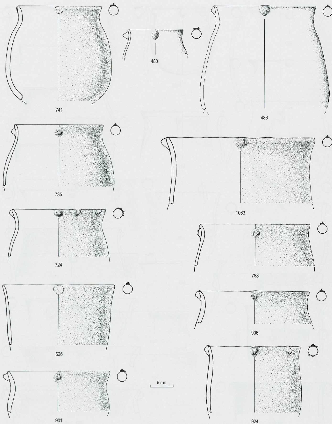
Planche 32. Ensemble E3B. Jarres à profil en S (type j10). Ech. 1 : 4.
