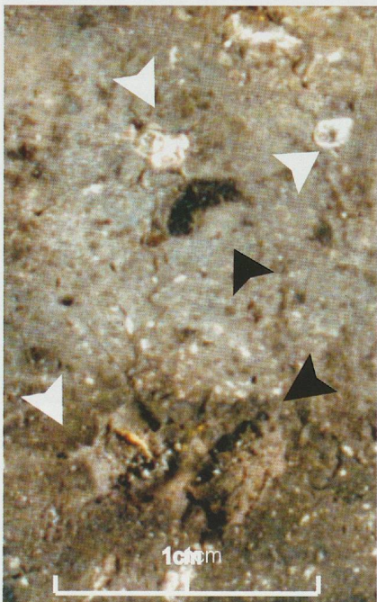
Planche 77d. Pâte à dégraissant calcaire coquillier : des débris de coquillages (flèches blanches) sont mêlés aux éléments calcaire. On voit aussi des cupules dues à la fusion du calcaire lors de la cuisson (flèches noires).
