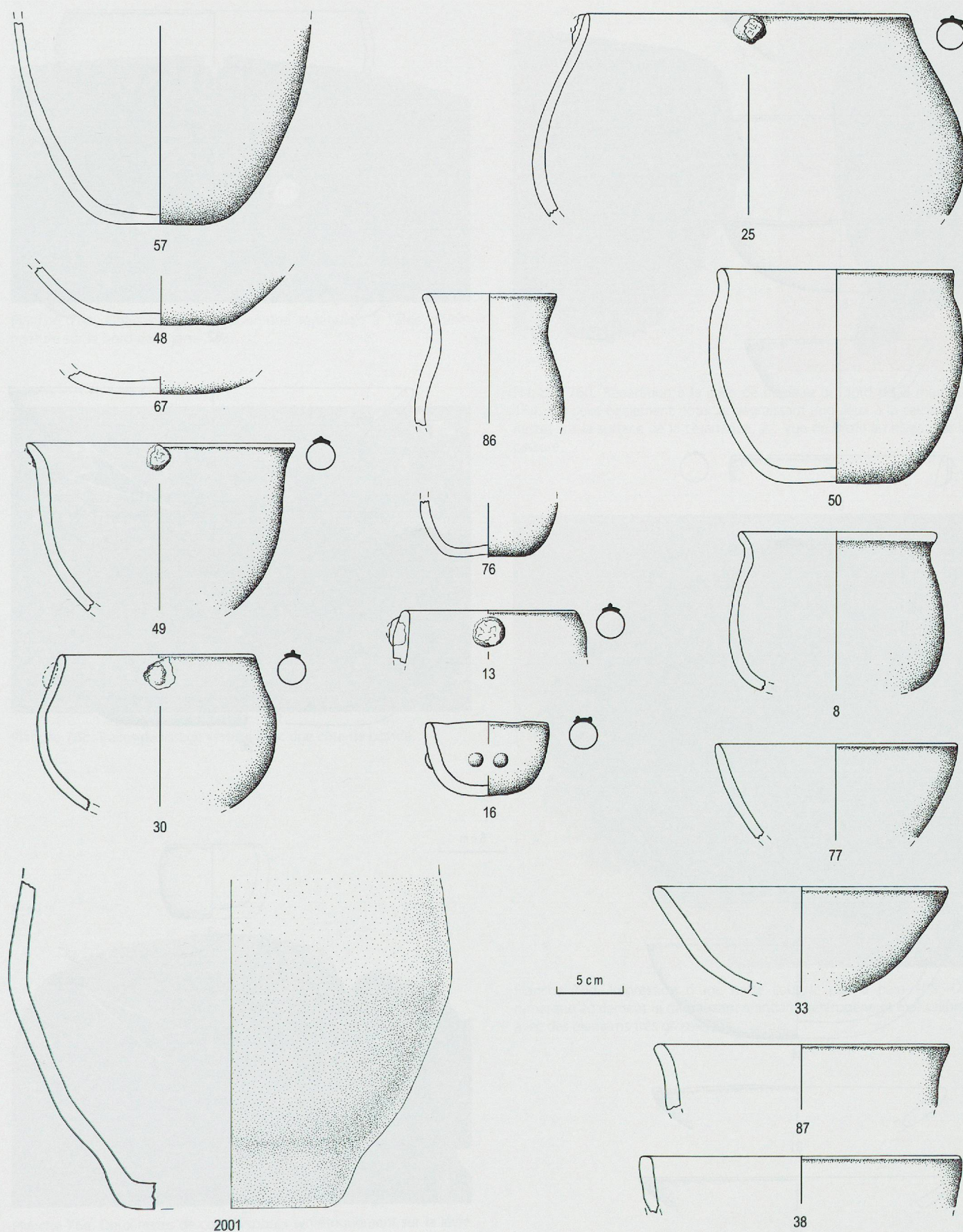
Planche 74. Ensemble E6. Jarres indéterminées. Gobelets (30, 76, 86). Marmites (8, 25, 49, 50). Bols (13, 16). Jatte (77). Grandes jattes (33, 38, 87). Ech. 1 : 4.
