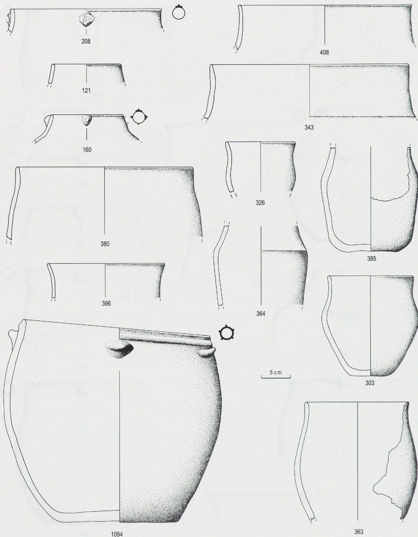
Planche 67. Ensemble E5. Jarres non segmentées à bord vertical (type j20 : 208, 380, 1094) ou rentrant (type j30 : 121, 160). Jarres segmentées à bord ouvert (type j40 : 303, 326, 396) ou vertical (type j50 : 343, 363, 364, 385, 408). Ech. 1 : 4.
