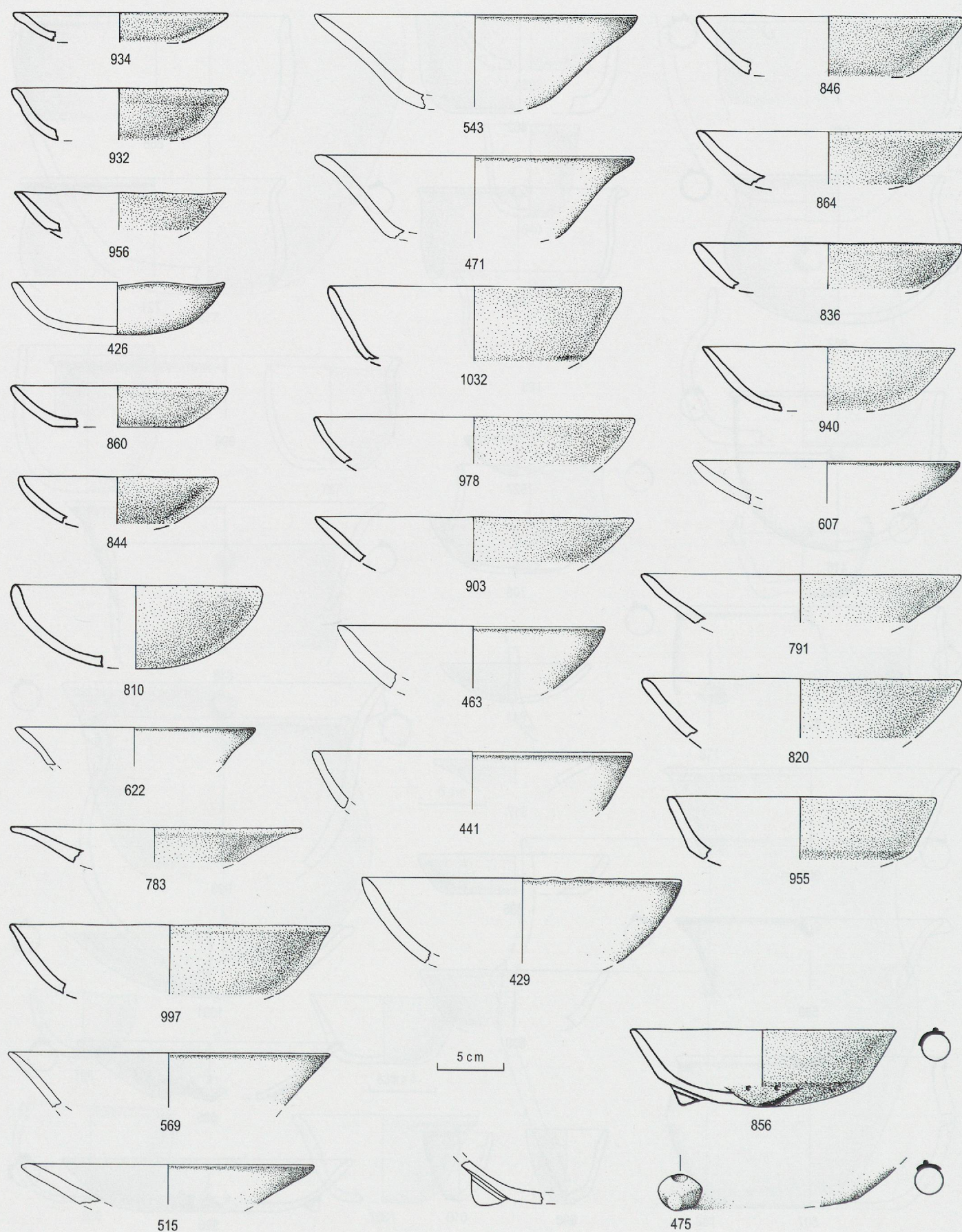
Planche 39. Ensemble E3B. Ecuelles (426, 622, 810, 844, 860, 932, 934, 956). Assiettes à bord éversé (type a10 : 471, 543, 569, 783, 997). Simples en V (type a11 : 515, 1032). Plat indéterminé. Ech. 1 : 4.
