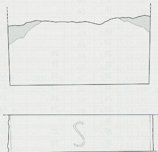
Fig. 269. Bloc d'assise cat. n° 538, en calcaire urgonien, avec une lettre S gravée. Ech. 1:20.
