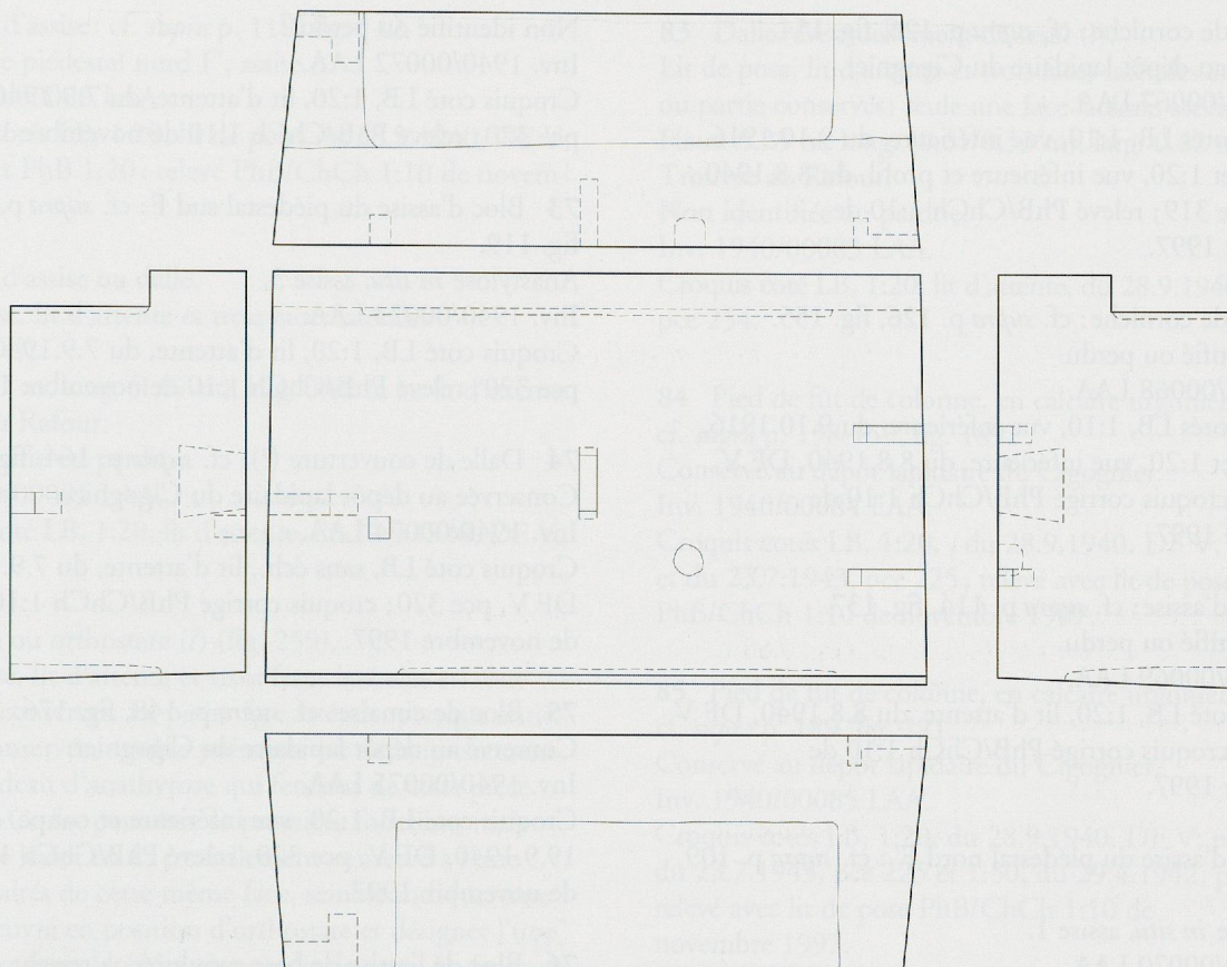
Fig. 256. Bloc d'assise cat. n° 61. Ech. 1:20.
