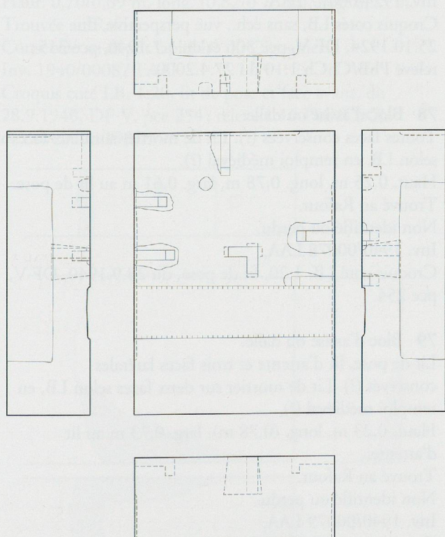
Fig. 257. Bloc d'assise cat. n° 64. Ech. 1:20.
