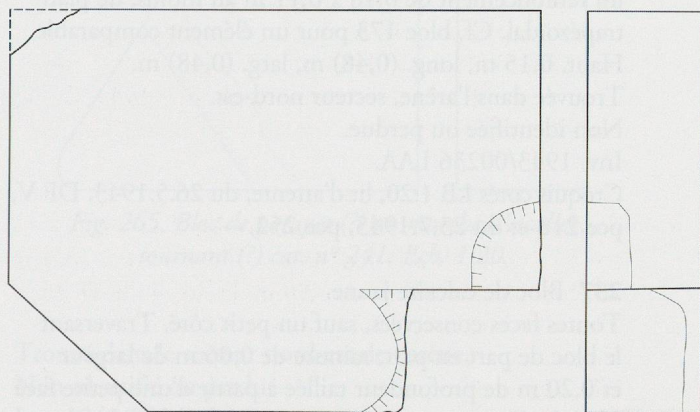
Fig. 263. Dalle de couverture du mur de podium cat. n° 218. Ech. 1:20.
