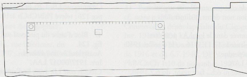
Fig. 255. Dalle de seuil cat. n° 55. Ech. 1:20.
