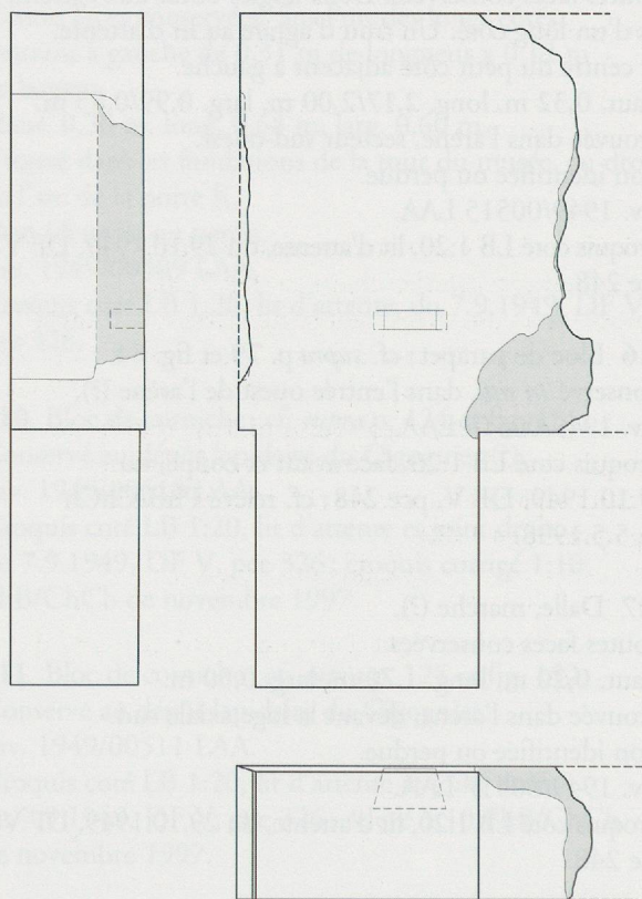
Fig. 266. Bloc d'assise à ressaut cat. n° 535. Ech. 1:20.
