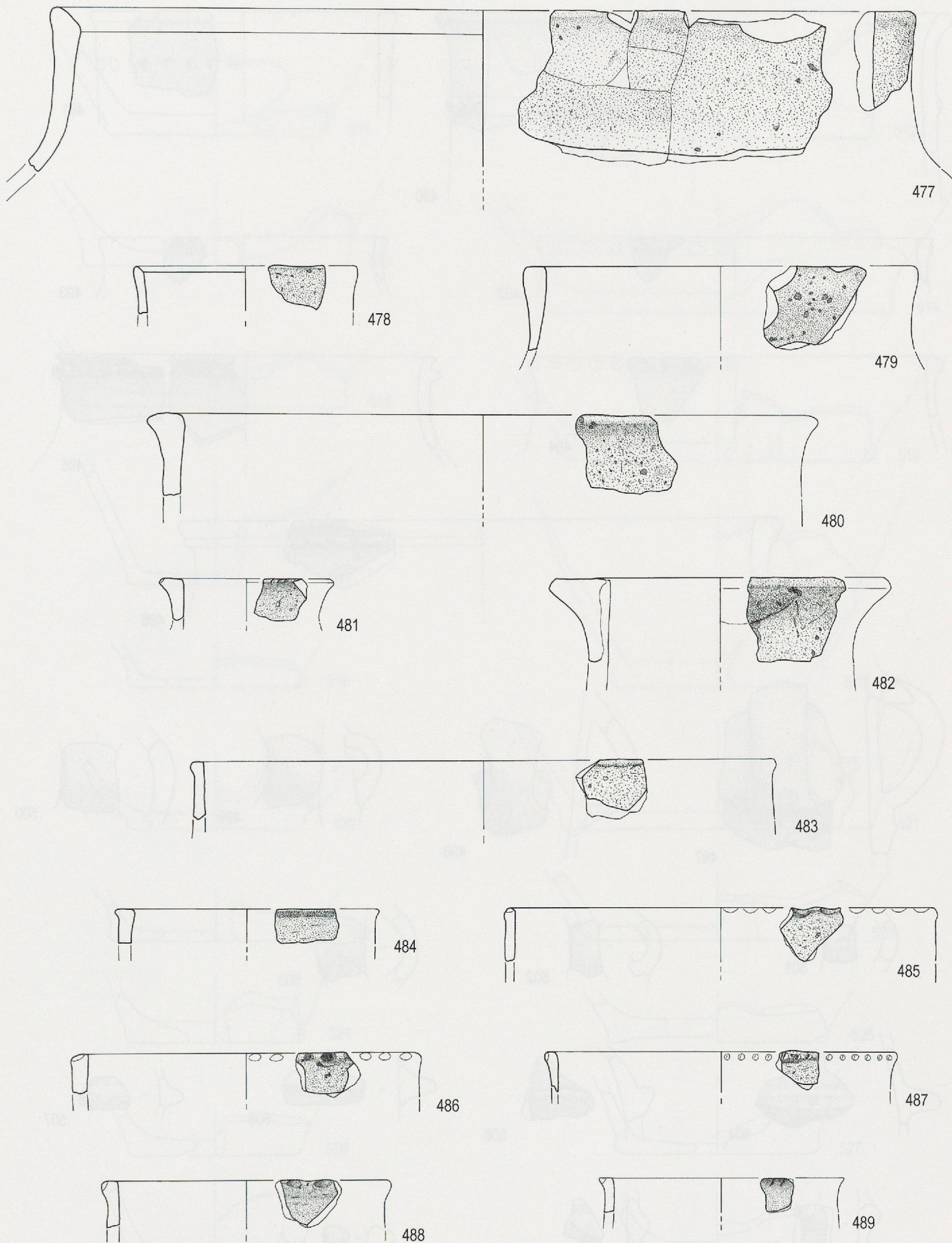
Pl. 39. Montricher VD Châtel d'Arruffens. Bronze moyen/récent. Cols cylindriques en céramique grossière (éch. 1:3).
