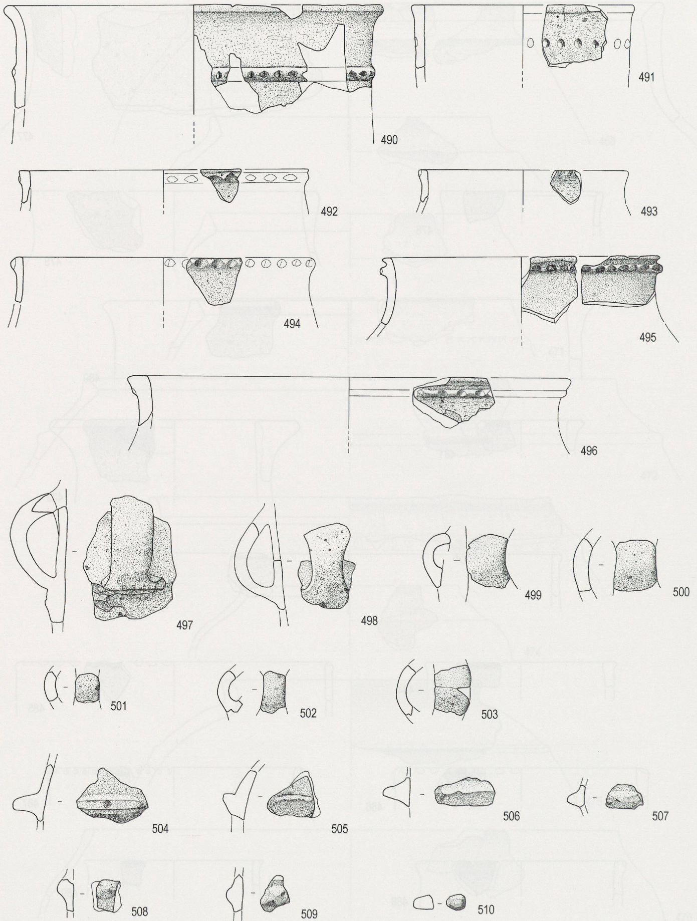
Pl. 40. Montricher VD Châtel d'Arruffens. Bronze moyen/récent. Cols cylindriques (490-496), anses (497-503), languettes (504-507) et mamelons (508-510) en céramique grossière (éch. 1:3).
