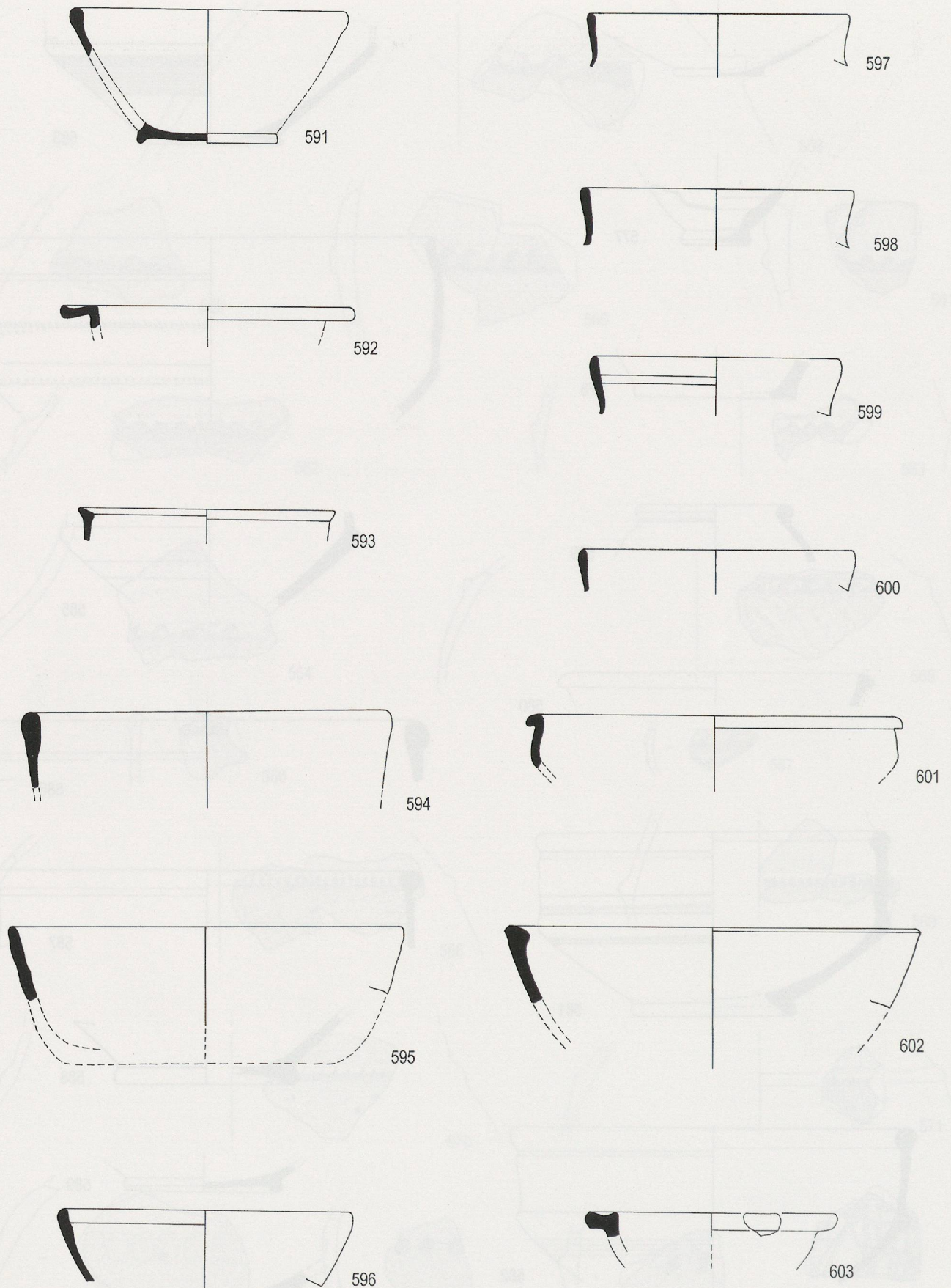
Pl. 46. Montricher VD Châtel d'Arruffens. Bas-Empire. Céramique à revêtement argileux (591-600) ; céramique sans revêtement apparent (601-603) (éch. 1:3).
