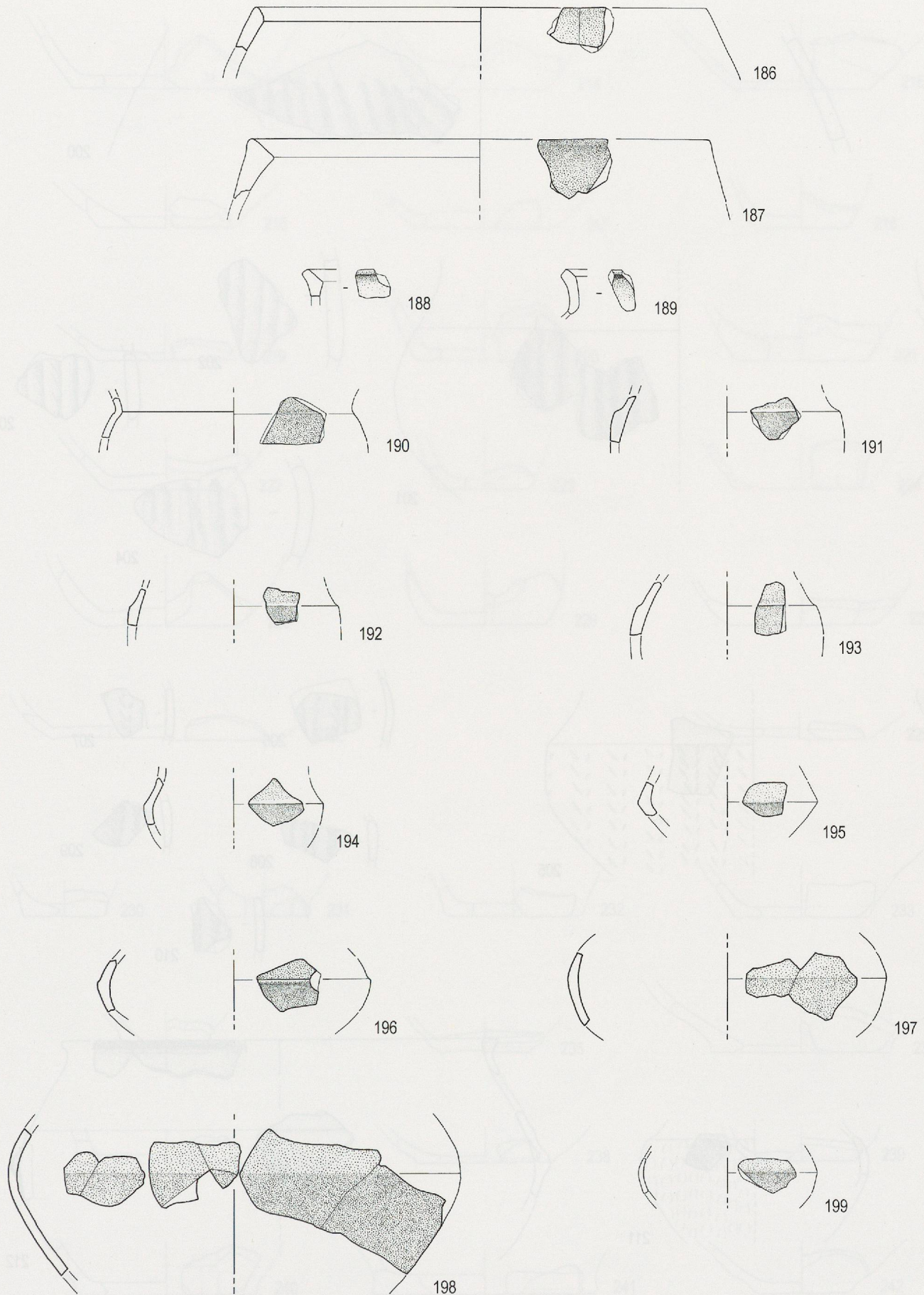
Pl. 19. Montricher VD Châtel d'Arruffens. Bronze moyen/récent. Corps à épaule rentrante sans encolure (186-187), lèvres segmentées (188-189), ressauts corps/col (190-194), corps biconiques (195-199) en céramique fine (éch. 1:3).
