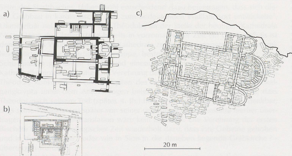
Abb. 91 Die drei Begräbniskirchen : a) Sion, St-Théodule (nach F.O. Dubuis/A. Antonini, provisorischer Plan, unpubliziert), b) St-Maurice, Sous-le-Bourg (nach Blondel 1953), c) Sion, Sous-le-Sceux
