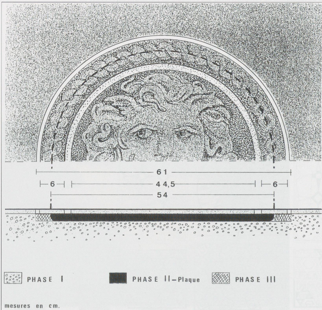
Fig. 10 - Schéma de mise en place de l'embléma (dessin M.-J. Schumacher - CEA)
