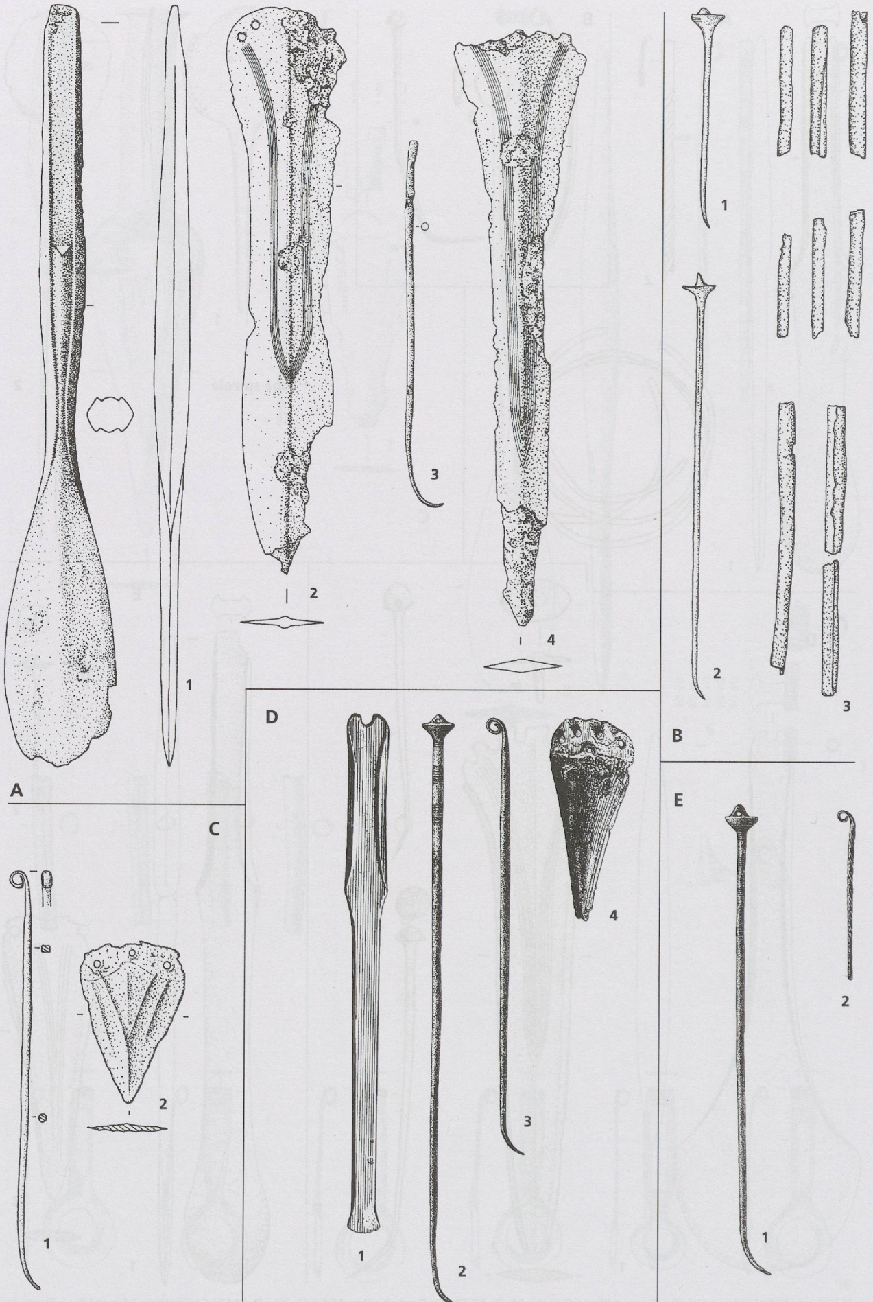
Pl. 21: A. [130] Villars-sous-Mont FR (d'après Abels 1972) ; B. [503] Jaberg BE Hinterer Jaberg (d'après Gallay 1971) ; C. [508] Enney FR Le Bugnon T.2 (d'après Gallay 1971) ; Spiez Einigen BE Holleweg, D. [475] T.1, E. [476] T.2 (d'après Grütter 1980) (éch. 1/2).
