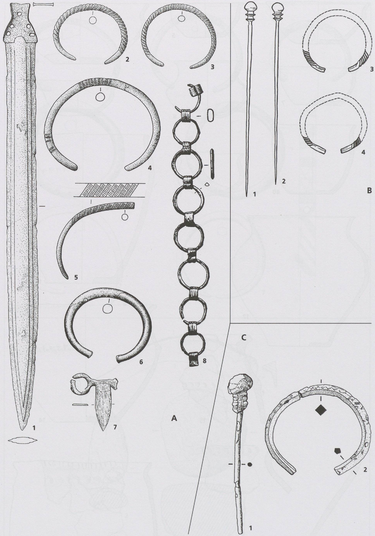
Pl. 47: A. [382] Sutz-Lattrigen BE (d'après Beck 1980 (1.7-8), Paszthory 1985 (2-6)); B. [512] Grenchen SO Breitenfeld (d'après Fey 1956) ; C. [449] Sion VS Rue de Lausanne (d'après Pugin 1984) (éch. 1/2).
