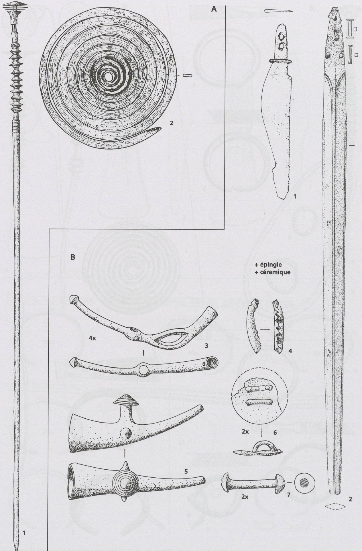
Pl. 39: A. [325] Bern BE Kirchenfeld (d'après Beck 1980); B. [1] Saint-Sulpice VD (d'après Schauer 1971 (1-2), Drack 1960-61 (3-7)) (éch. 1/2).
