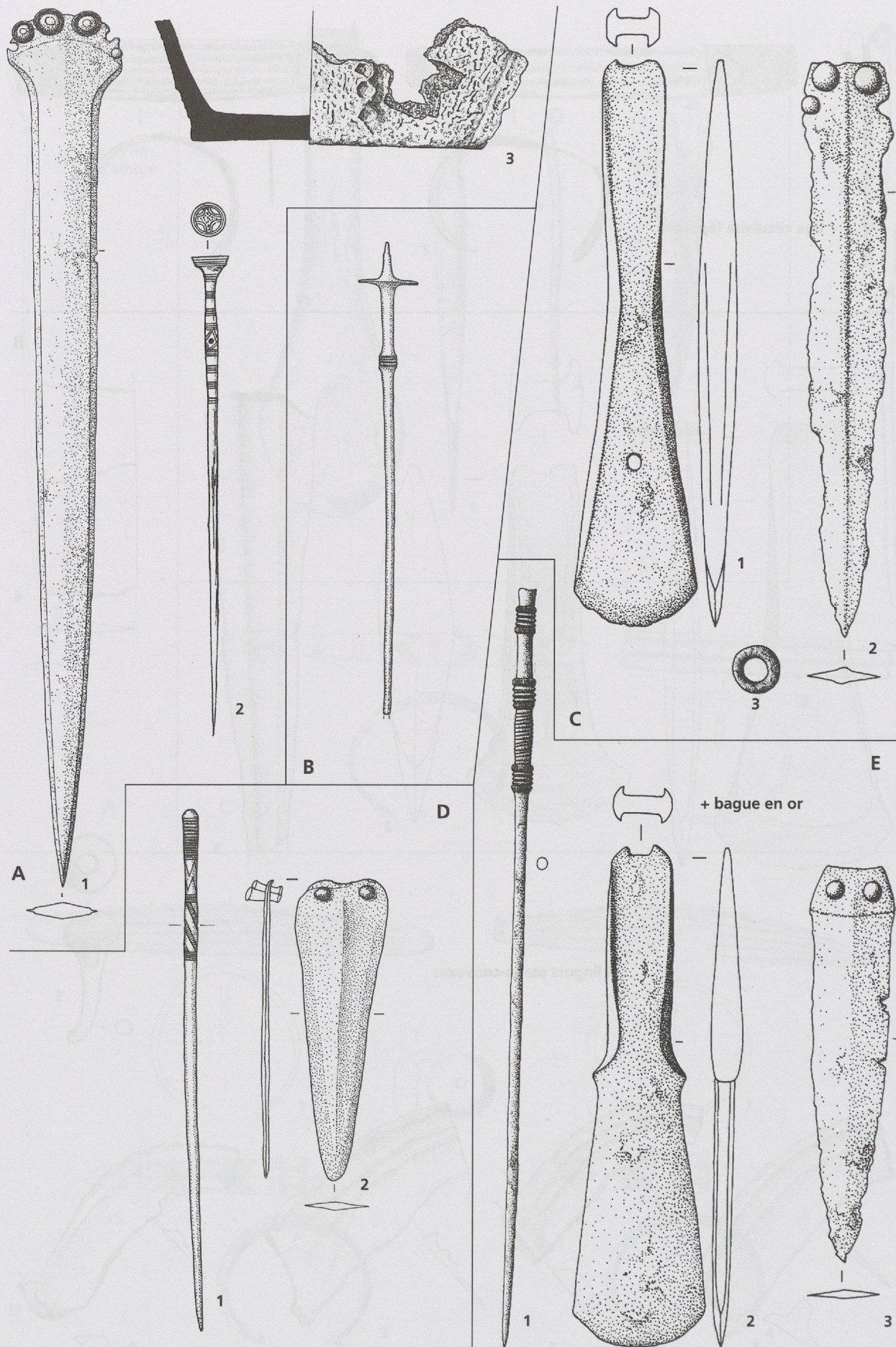
Pl. 29: A. [6] Ollon Saint-Triphon VD Le Lessus «tombe du guerrier» (d'après Schauer 1971 (1), Bocksberger 1964 (2-3)) ; Neueneegg BE Im Forst, B. [361] T.2, D. [355] T.1; C. [65] Veytaux VD Chillon (d'après Abels 1972) ; E. [29] Cressier NE La Baraque (d'après Abels 1972) (éch. 1/2, sauf A, 1 1/3).
