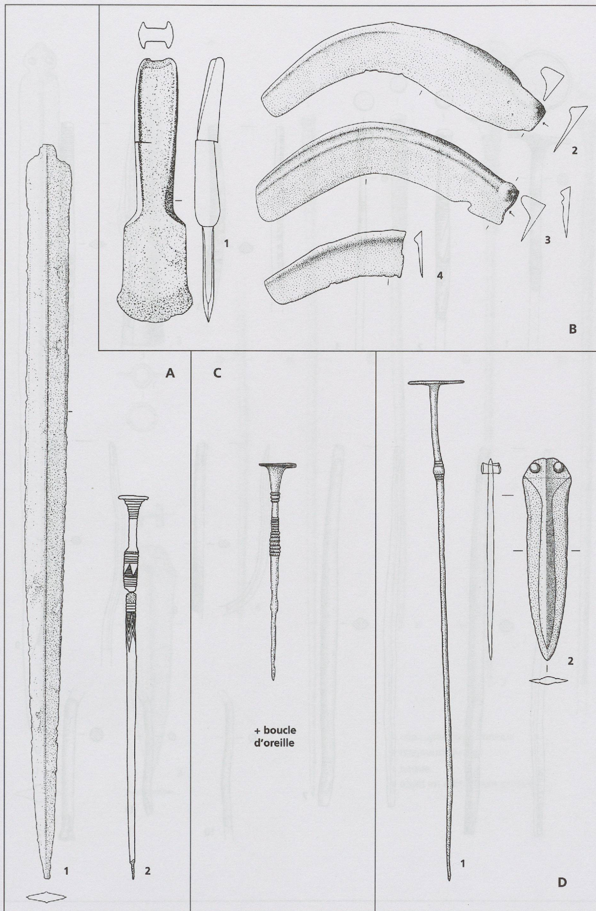
Pl. 32: Gals BE Jolimont, A. [360] T.4 (d'après Schauer 1971 (1), Osterwalder 1971 (2)), C. [530] T.1; B. [69] Vouvry VS Dans les vignes (d'après Abels 1972 (1), Primas 1986 (2-4)) ; D. [2] Ollon Saint-Triphon VD Tombe Gaudard (éch. 1/2, sauf A, 1 1/3).
