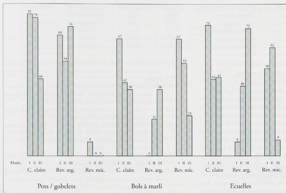
Fig. 327. Avanches-En Chaplix. Matériel en structures (matériel d'attribution sûre ou probable).
