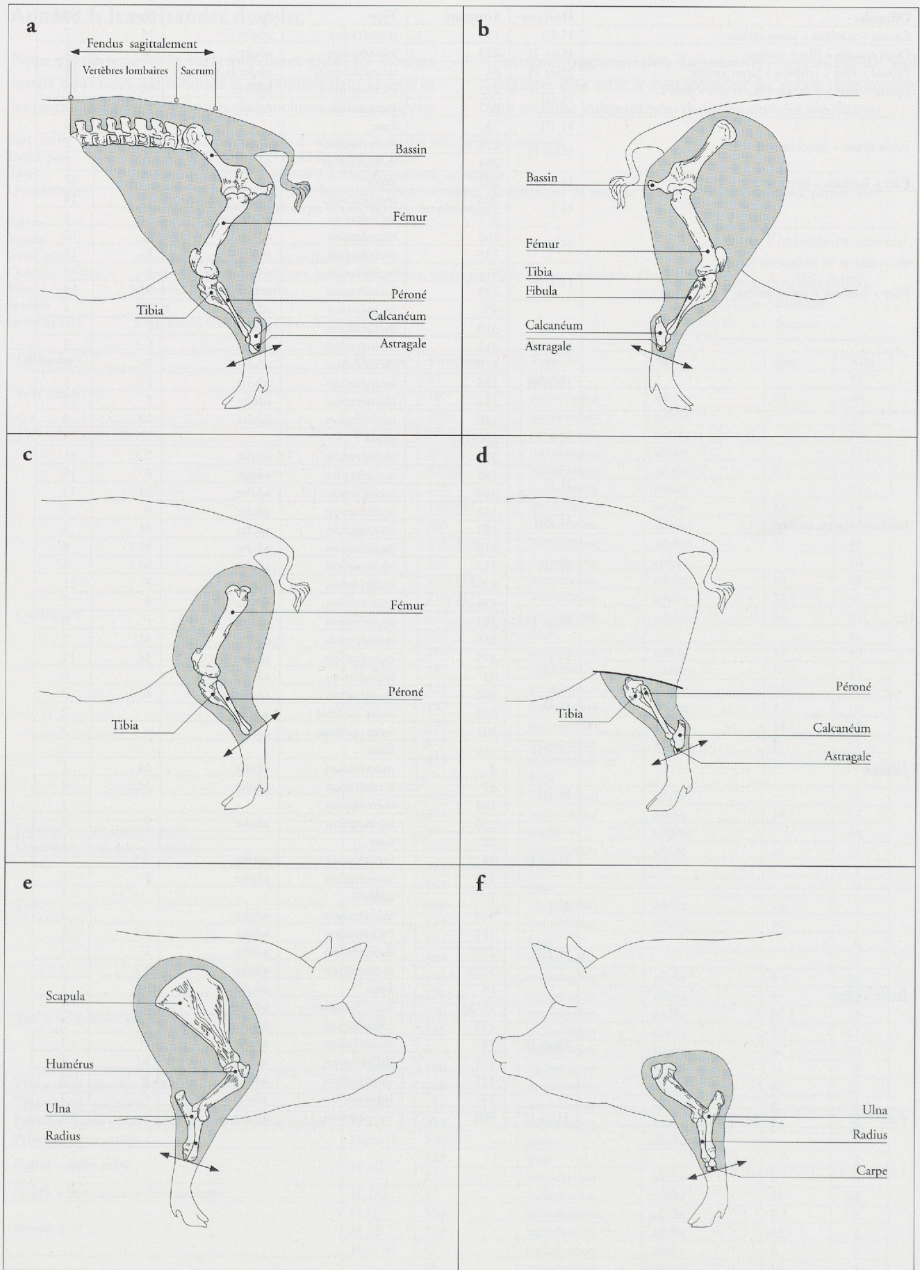
Fig. 170. Avenches-En Chaplix. Quelques exemples d'offrandes de porc. Correspondance des quartiers de viande et des portions squelettiques. a: quartier arrière; b: filet, jambon et jarret arrière; c: jambon et jarret arrière; d: jarret arrière; e: palette, épaule et jarret avant; f: épaule et jarret avant.
