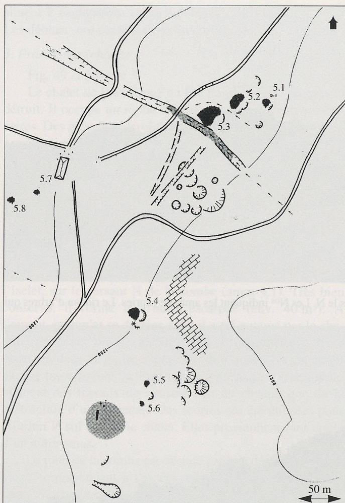
Fig. 55. Schéma du site des Convers (Saint-Blaise, 74, F). 1:5000.
