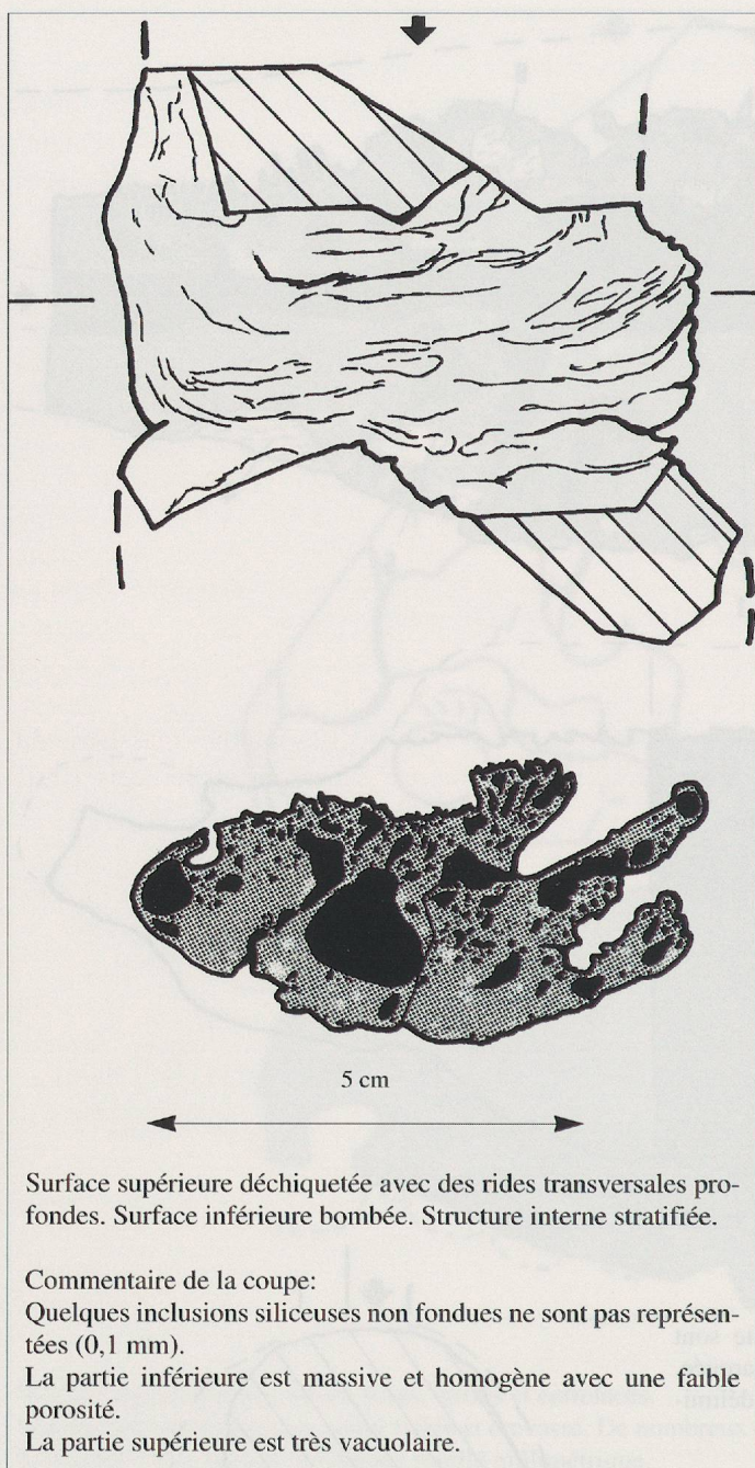
Fig. 73. Scorie coulée grise à texture vacuolaire, coulure épaisse en canal: Ech. SLF 41 (Salève, Rochers de Faverges, amas 17.1).
