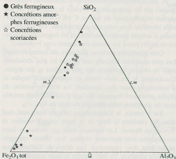
Fig. 46. Composition chimique du Sidérolithique du Salève.
