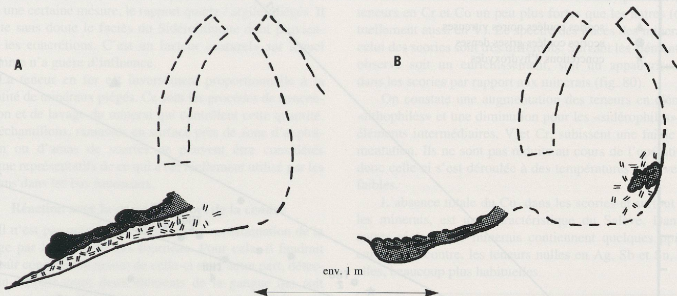
Fig. 77. Schéma des deux techniques de réduction du Salève. A: bas fourneau à scories coulées noires vitreuses (SVN). B: bas fourneau à scories coulées grises denses (SGD).
