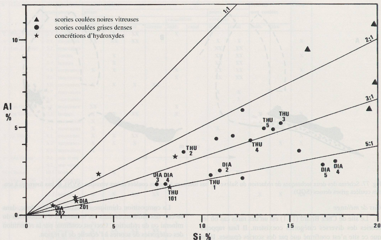
Fig. 78. Rapport Si:Al des échantillons du Salève.
