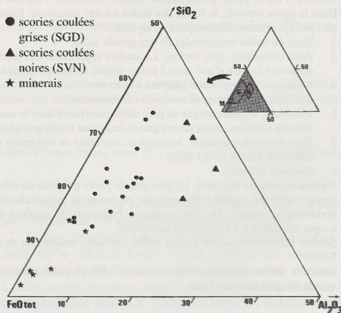
Fig. 74. Composition chimique des scories du Salève.
