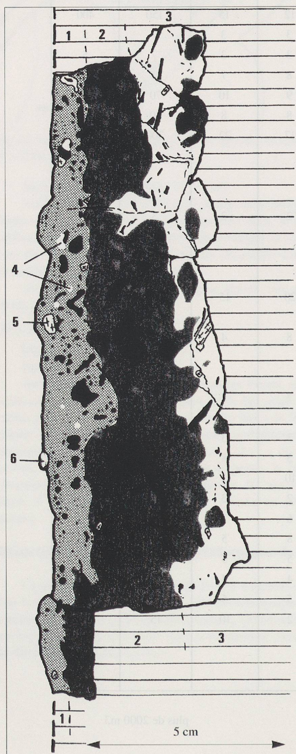
Fig. 67. Fragment de revêtement interne d'un fourneau. Ech. SLP 51 (Le Pommier, site 12, amas 12.2, Salève). Vue en coupe.
