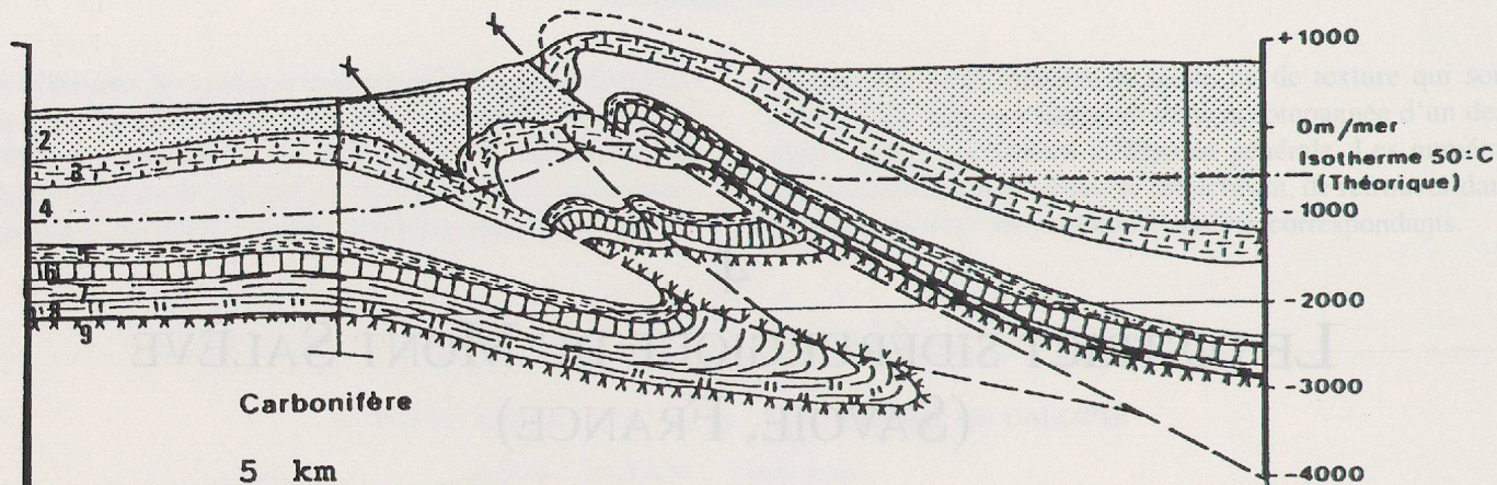
Fig. 43. Profil géologique schématique à travers le Salève et les terrains adjacents. Extrait du profil géologique schématique du canton de Genève (Amberger, 1982, p.24-25). Echelle 1:100 000
