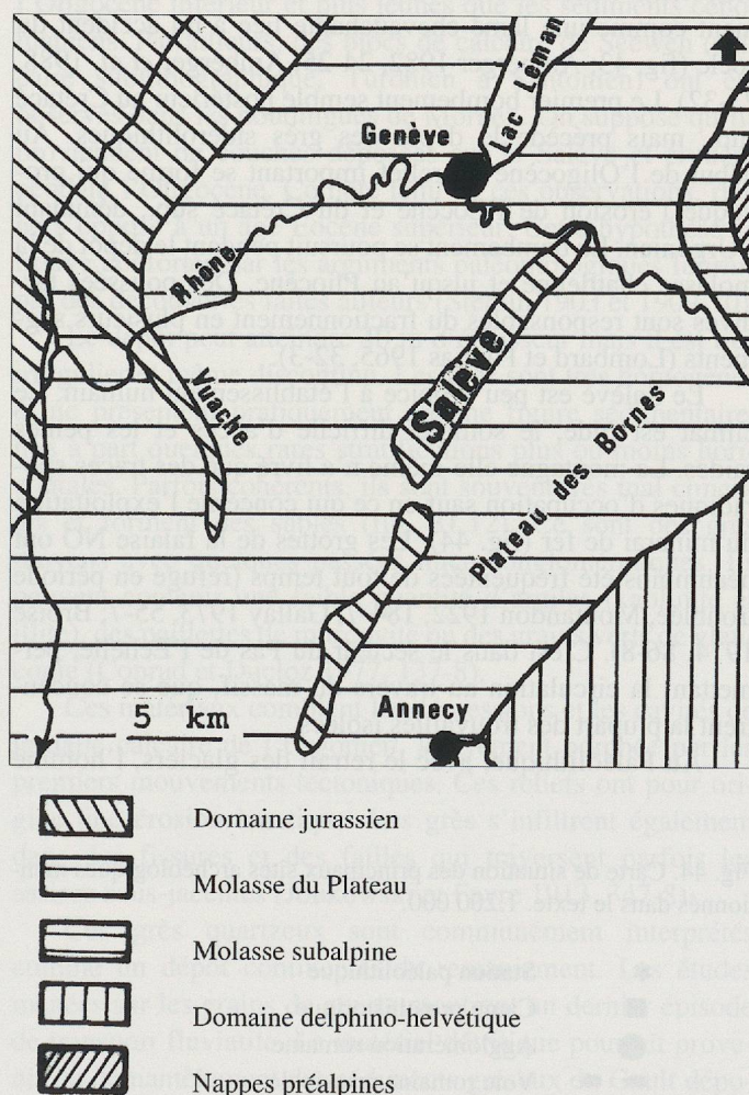
Fig. 42. Carte tectonique simplifiée du Salève.
