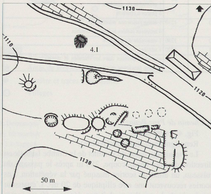
Fig. 51. Schéma du site de L'Iselet (Cruseilles, 74, Fr.). 1:2500.
