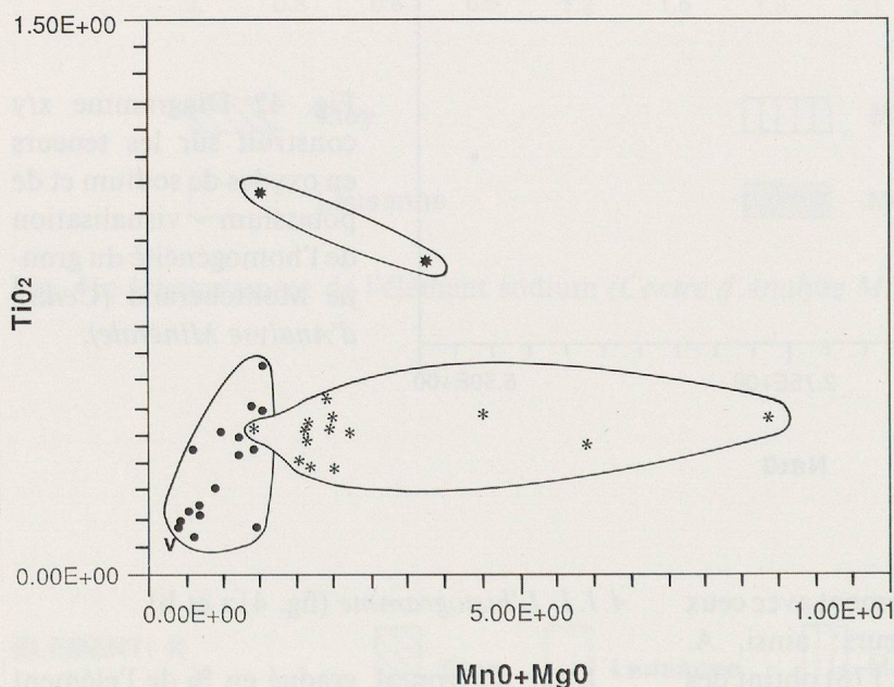
Fig. 43 Diagramme x/y construit sur la teneur en \text{TiO}_2 et sur la somme des teneurs en \text{MnO} et \text{MgO} - discrimination des sites de provenance (Centre d'Analyse Minérale).
