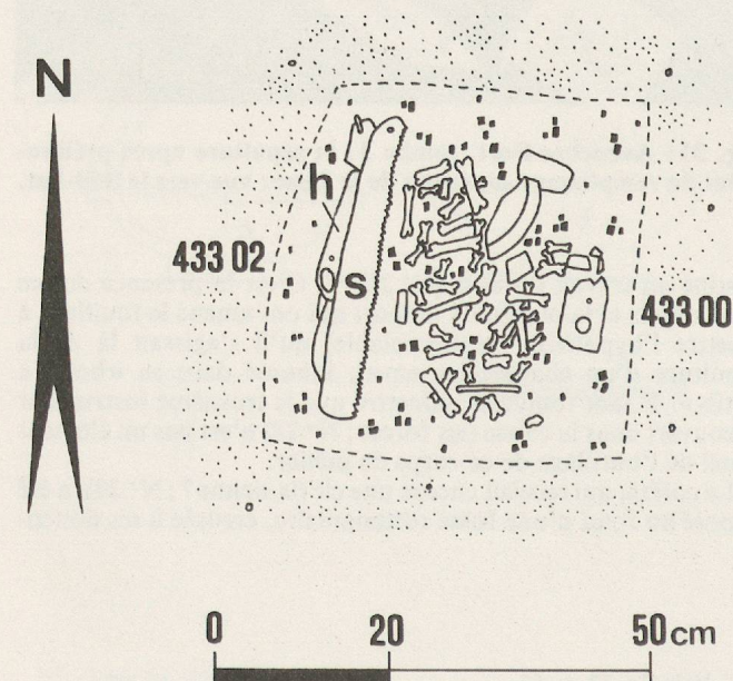
Fig. 32: Avenches-Port, tombe 3: plan de la partie inférieure de la sépulture (s = scie; h = herminette).
