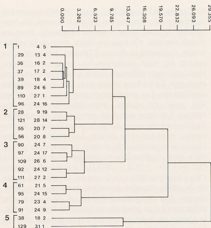
Fig. 7 Auvernier/Nord. Compositions chimiques aberrantes en arsenic, antimoine, nickel et cobalt. Dendrogramme de la classification hiérarchique ascendante. Distance: carré de la distance euclidienne, agrégation: chaînage complet.
