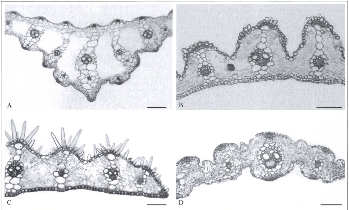
Fig. 1. – Cortes transversales. A. Sacciolepis vilvroides (Hook 1157A); B. S. chevalieri (Laegaard 16223); C. S. ciliocincta (Adams 15121); D. S. striata (Kearney 1618). [Barra: A = 200 µm; B, C y D = 100 µm]
