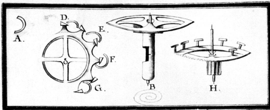
Description de l'Escapement de M r Graham, Horloger Anglois; Le dit Escapement à Répète, vulgairement dit à Cylindre
