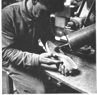
Ein Korkboden erhält den letzten Schliff.
