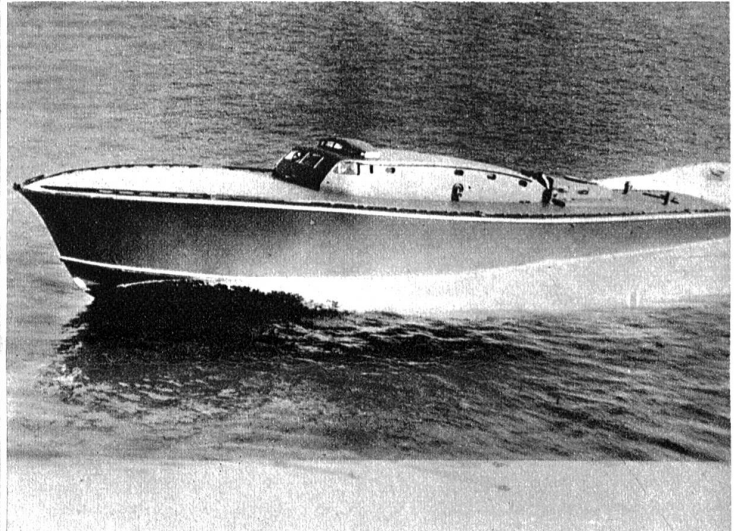
Englands modernstes Torpedoschnellboot. Das 25 Meter lange Boot entwickelt mit seinen drei 1000 PS Rolls Royce-Motoren eine Geschwindigkeit von 92,755 Stundenkm. Es ist ausgerüstet mit zwei Torpedorohren v. 53 cm od. mit 4 Torpedorohren von 45,70 cm Kaliber, Kanonen, Tiefseebomben und Verneblungsapparaten. Associated Press
