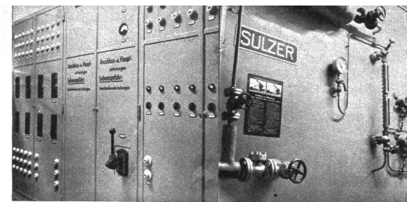
Elektro-Dampfkessel mit Verteilerraum und Kondensgefäss
