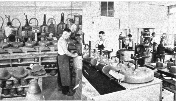
Dressieren und Pressen der Hüte
