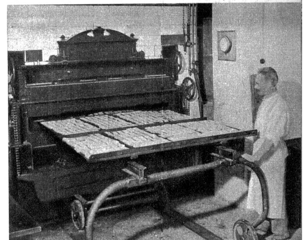
Zwiebackröstofen
