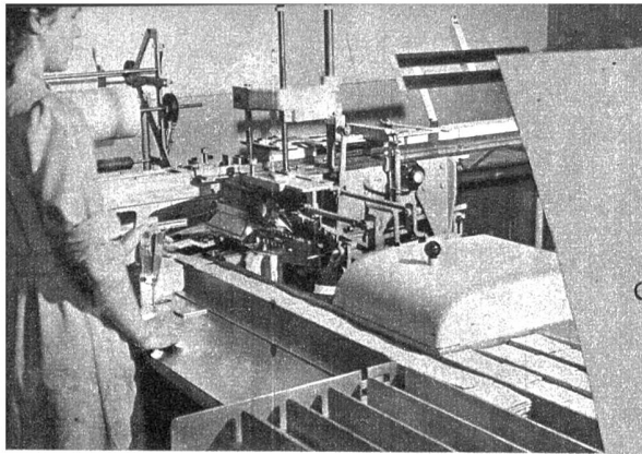
Hier werden pro Minute 40 Pakete Dar-Vida gewickelt
