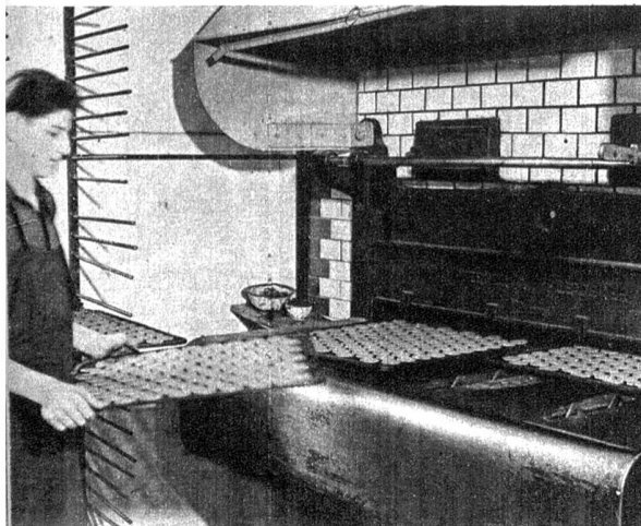
Nach 7 Minuten kommen die Biscuits am andern Ende gebacken heraus
