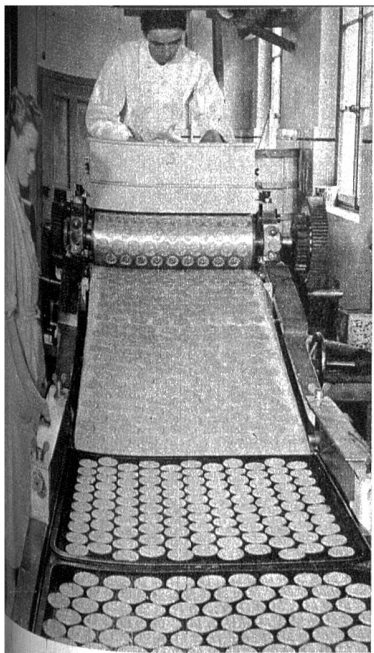
Gebäckformmaschine
