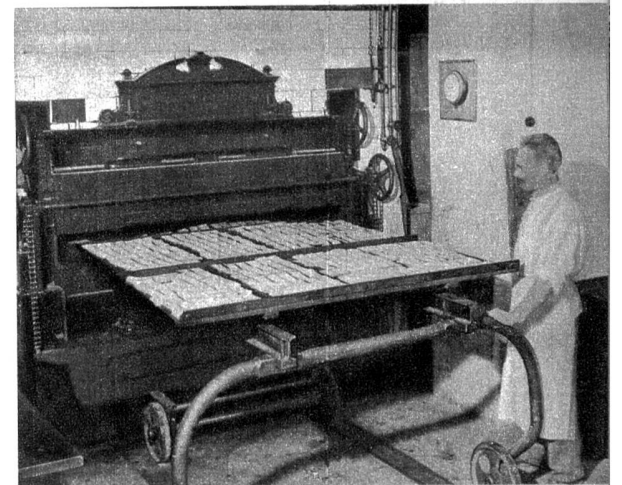
Zwiebackröstofen
