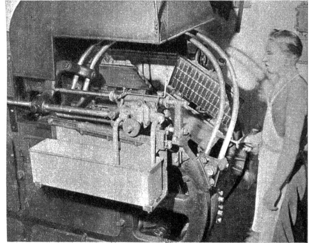
Waffelbackofen mit Gasfeuerung
