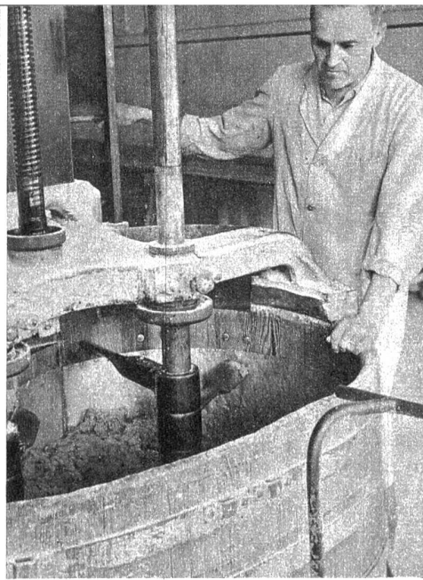
Knetmaschine für 280 kg Mehl
