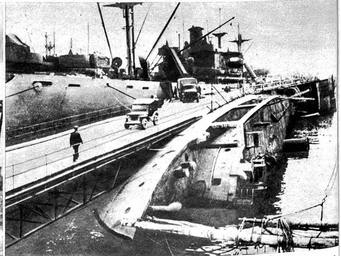
Im Hafen von Neapel haben amerikanische Pioniere auf einem umgekippten Transportdampfer eine Landebrücke gebaut. Auf diese Weise können die Nachschubschiffe neben dem mit Schlagseite auf Grund liegenden Schiff gelöscht und der Hafen seinem Zwecke nutzbar gemacht werden
