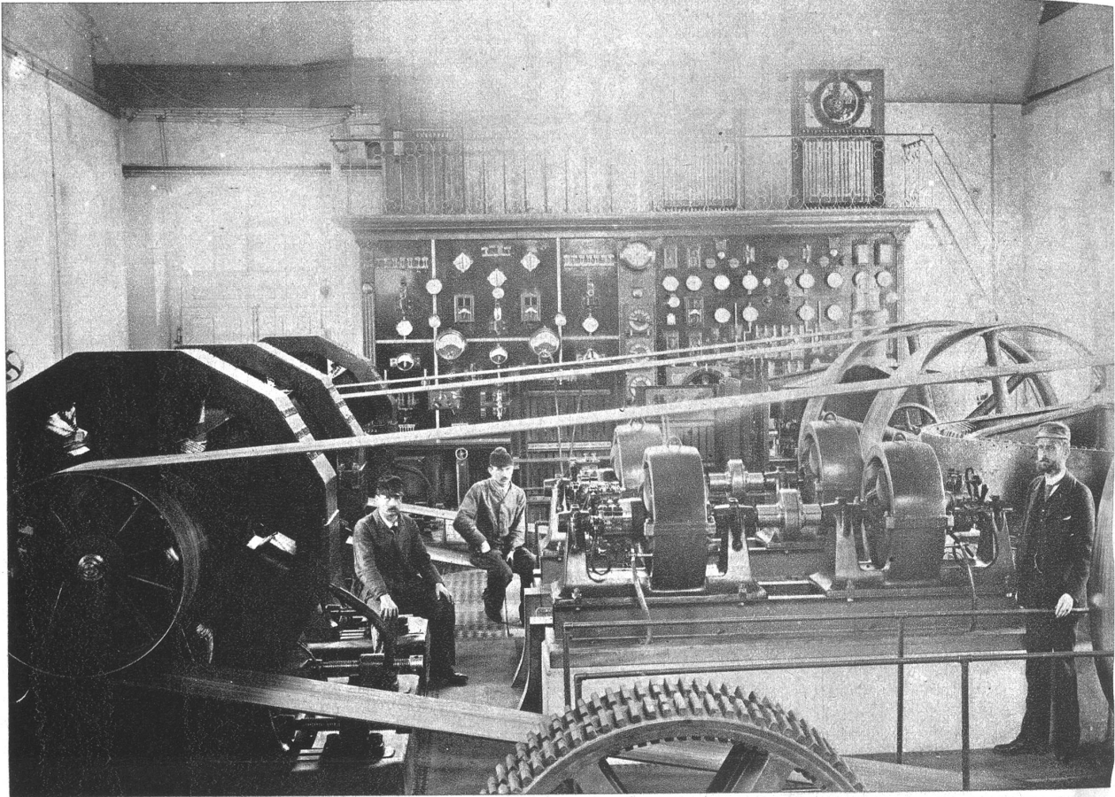
Innenaufnahme aus dem ersten Elektrizitätswerk der Stadt Bern. (Siehe Artikel auf Seite 852 unten.)
