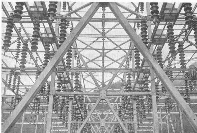
Stromluftstation Innertkirchen. Transformatorenanlage.
