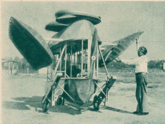
Ein «Insekten-Flugzeug» will ein kalifornischer Erfinder, Harry Cordy, konstruieren. Beim Aufsteigen sollen die Flügel eingezogen und beim Landen wieder entfaltet werden.
