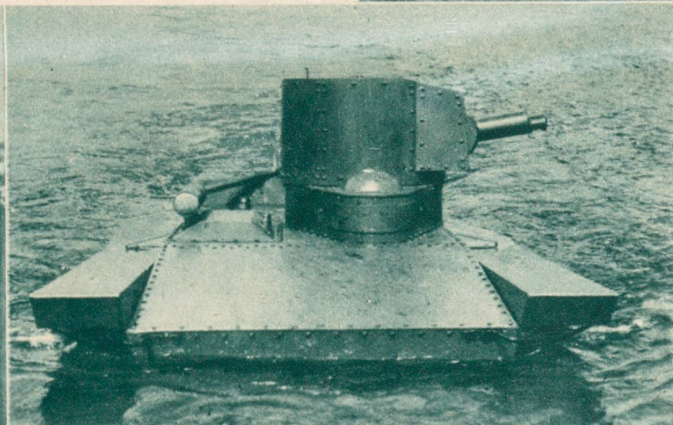
Ein schwimmender Tank
