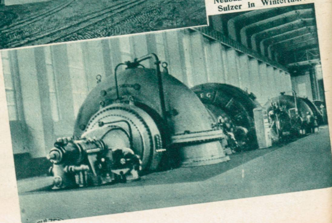
Rechts: Speicher- Kraftwerk Herdecke (Deutschland), aus- gerüstet mit drei Sulzer-Speicher- pumpen von je 12,300 Liter pro Se- kunde, 163 Meter Förderhöhe und 33,000 Pferdestär- ken Kraftbedarf. Phot. Gebr. Sulzer A.-G., Winterthur.
