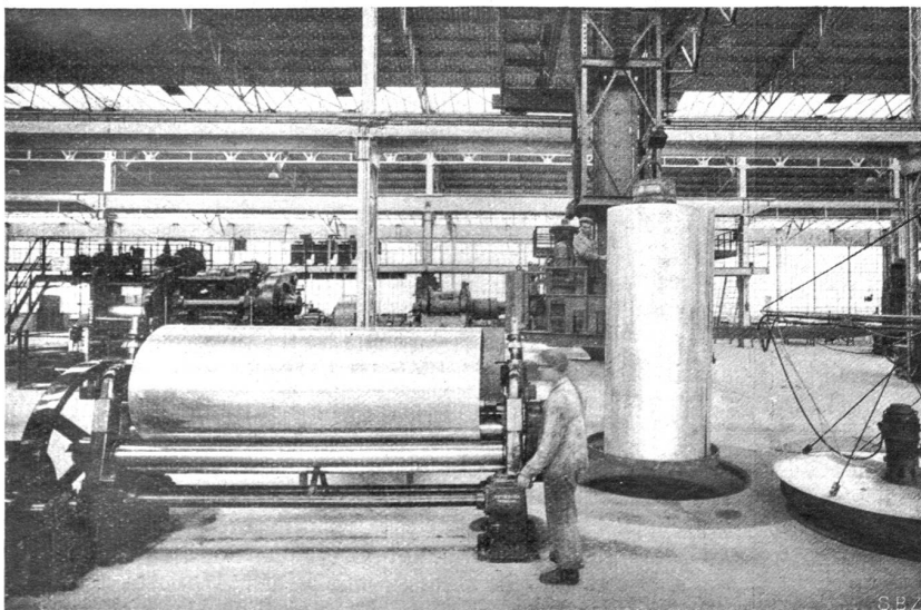
Aluminiumwerke in Chippis. — Einrollmaschine für Bleche, rechts Topf.
