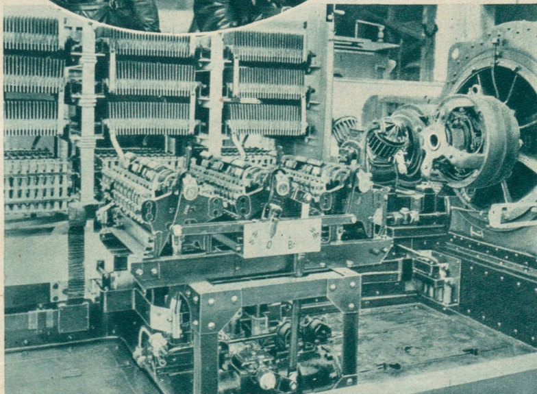
Im Innern einer elektrischen Lokomotive. Photo Sécheron.
